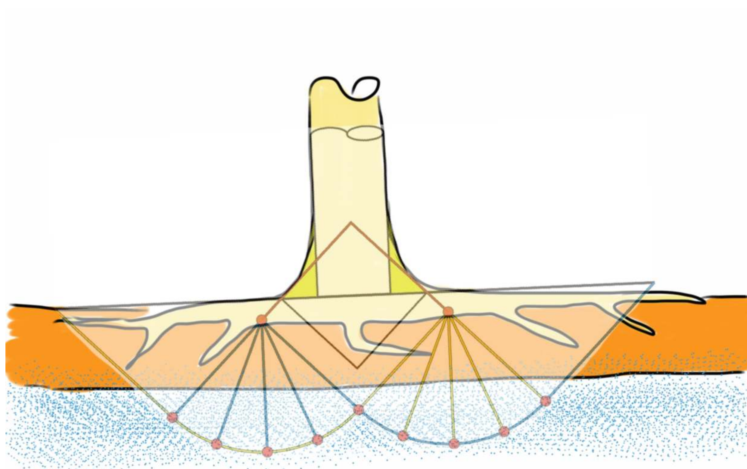
Staunässe
