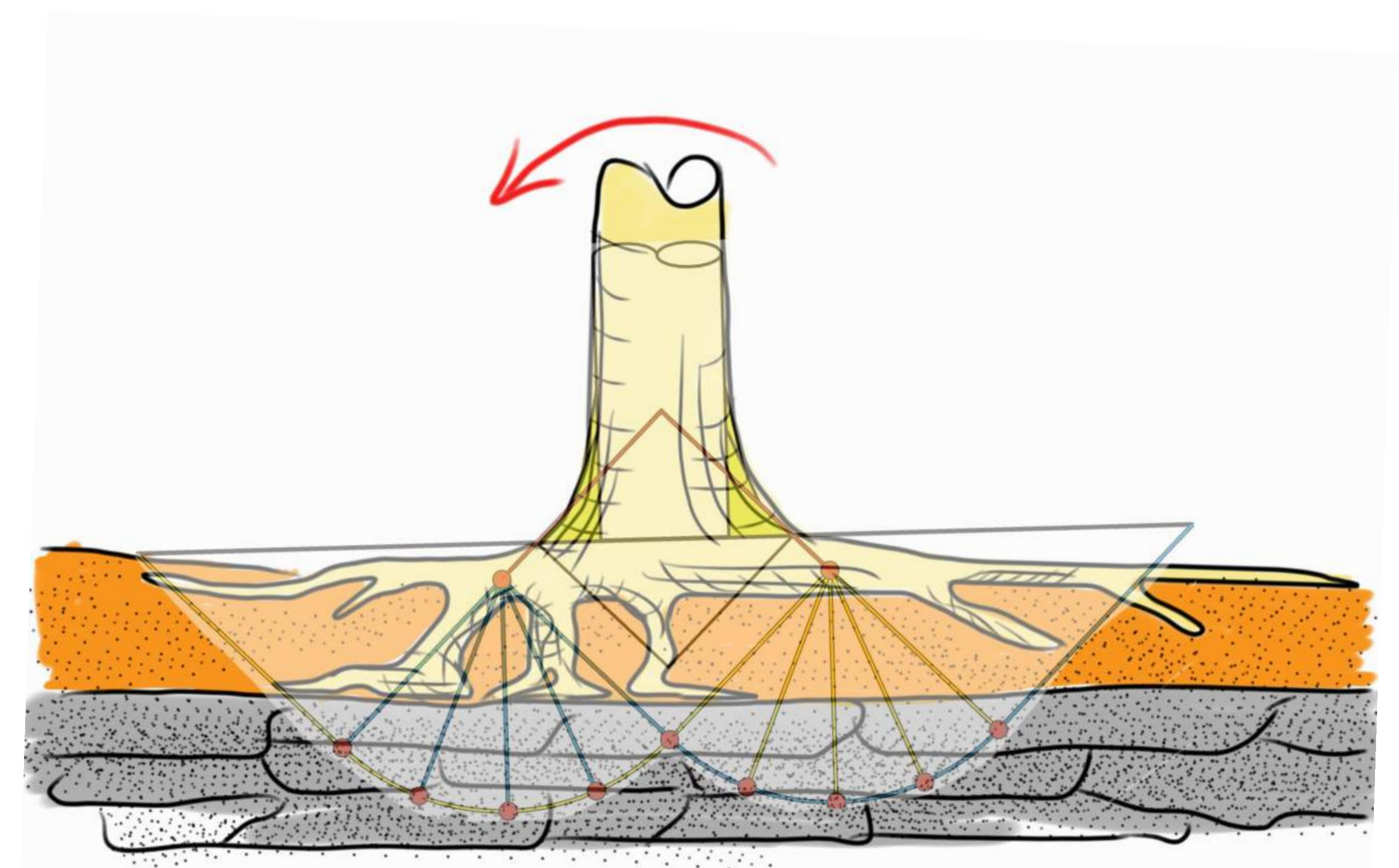
Felsengrund
