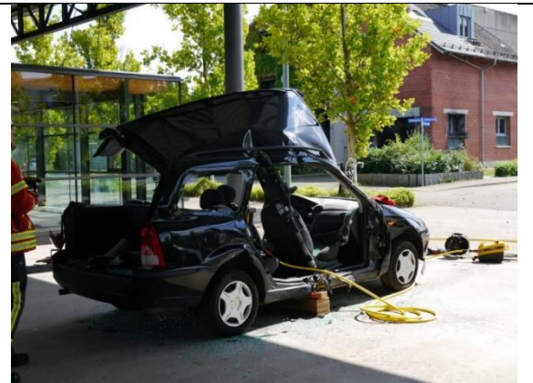
Abbildung 43: Arbeiten mit dem Rettungszyylinder - Versuchsfahrzeug 2
