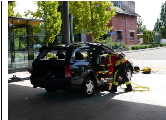
Abbildung 42: Arbeiten mit dem Rettungszyylinder - Versuchsfahrzeug 2
