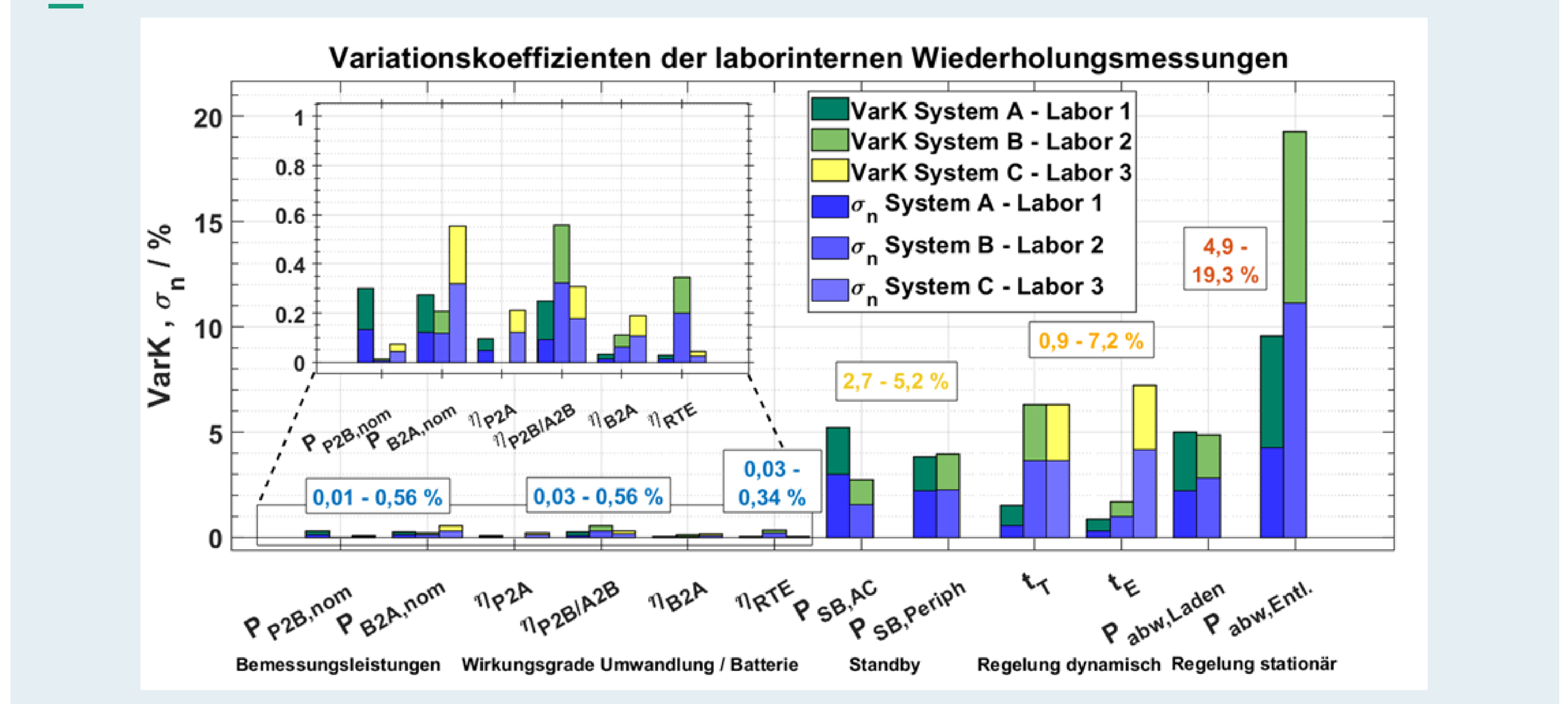
Abbildung 1 Laborinterne Wiederholbarkeiten aus den Erstvermessungen für verschiedene Systemtopologien
