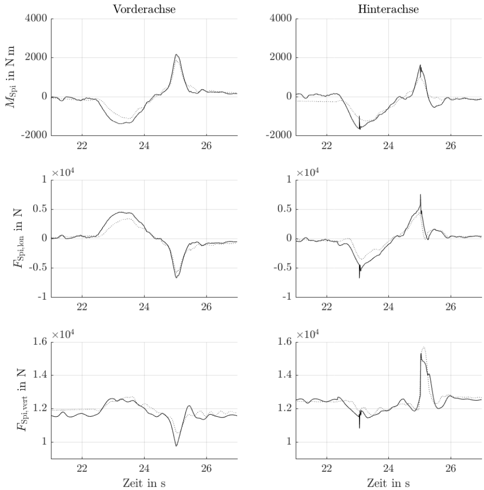
Abbildung C.12: Messung #629
