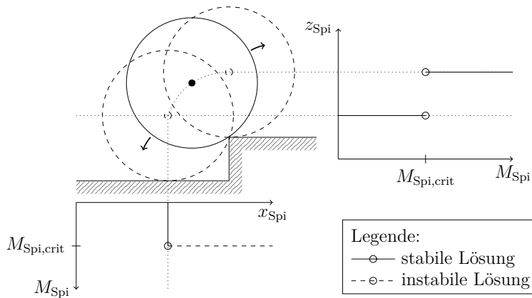
Abbildung 3.11: Die Lösungen für die (x_{\text{Spi}}, z_{\text{Spi}}) Position eines starren Rades an einem stufenförmigen Hindernis in Abhängigkeit des Drehmoments am Radmittelpunkt M_{\text{Spi}} unter der Annahme konstanter F_{\text{Spi,lon}} und F_{\text{Spi,vert}} .
