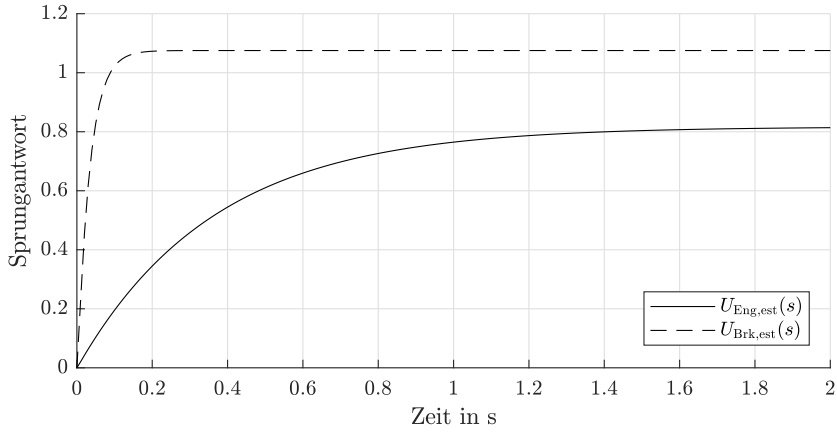
Abbildung C.20: Die Sprungantworten der identifizierten PT2-Modelle U_{Eng,est}(s) und U_{Brk,est}(s) .
