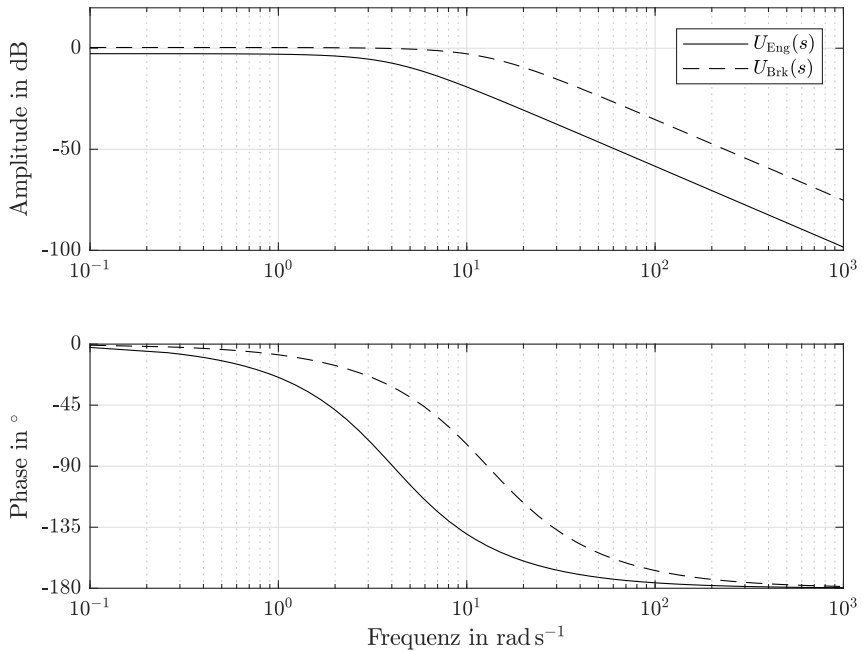
Abbildung C.19: Die Bodediagramme der identifizierten PT2-Modelle U_{\text{Eng}}(s) und U_{\text{Brk}}(s) .
