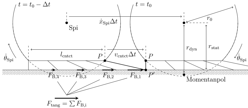
Abbildung 3.3: Veranschaulichung des Bürstenmodells anhand eines angetriebenen Rades zu zwei Zeitpunkten. Mithilfe dicker Linien ist das Bürstenelement am Punkt P des Reifens hervorgehoben, welches in die Kontaktfläche zum Zeitpunkt t_0 - \Delta t eintritt und sie zum Zeitpunkt t_0 wieder verlässt. Sein Kontaktpunkt P' mit der Fahrbahn bleibt dabei stets derselbe.
