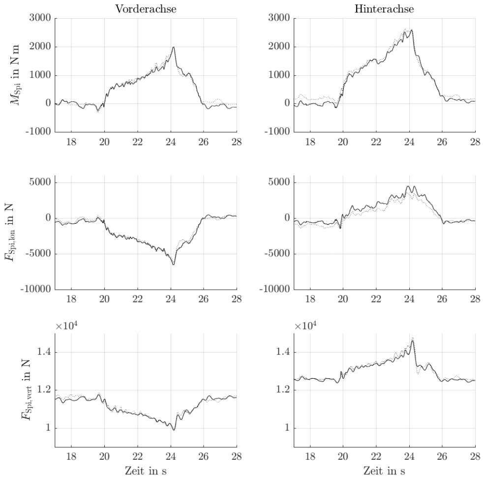
Abbildung C.1: Messung #481
