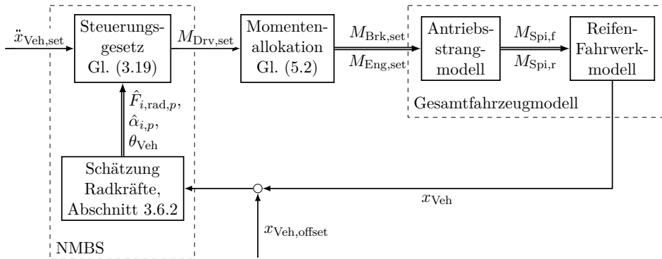
Abbildung 3.24: Blockschaltbild für die Simulation der NMBS mit der Möglichkeit zur Manipulation der in der NMBS angenommenen Längsposition des Fahrzeugs durch x_{\text{Veh,offset}} .
