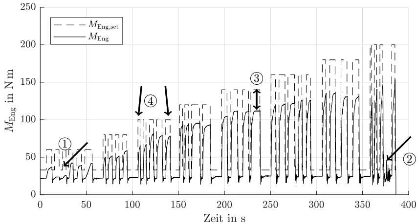
Abbildung 4.5: Aneinandergereihte Einzelmessungen mit Sollwertsprüngen für das Antriebssystem.
