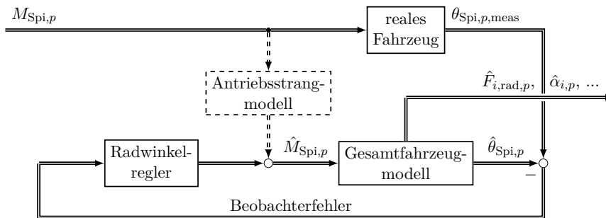
Abbildung 3.21: Signalflussdiagramm einer Struktur zur Schätzung der modellinternen Größen. Fallen die Eingangsgrößen M_{Spi,p} weg (gestrichelter Teil), so wird der Beobachter zum UIO.
