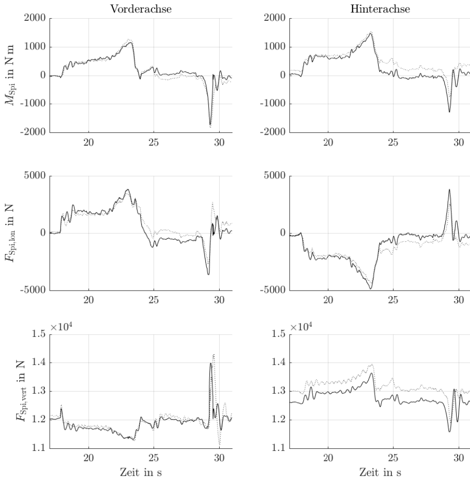
Abbildung C.3: Messung #673
