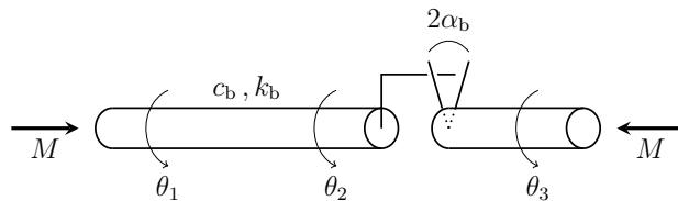
Abbildung A.3: Ein einfaches Modell für Spiel und Elastizität in Anlehnung an [LE07].
