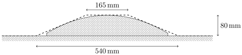
(d) Bremsschwelle mit einem Kreissegment als Querschnitt.
