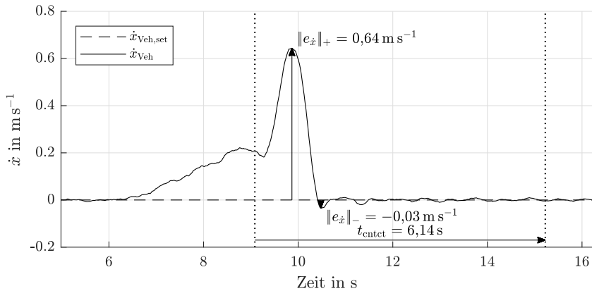
(b) Geschwindigkeitsverlauf
