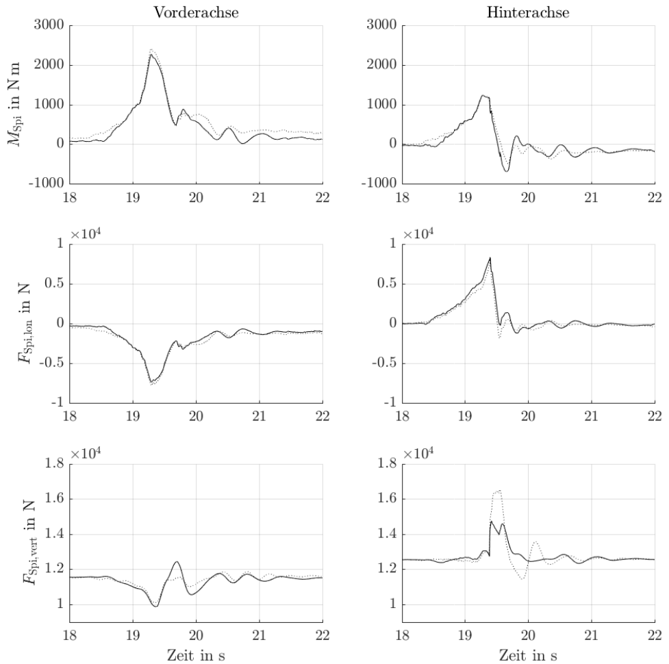
Abbildung C.2: Messung #482
