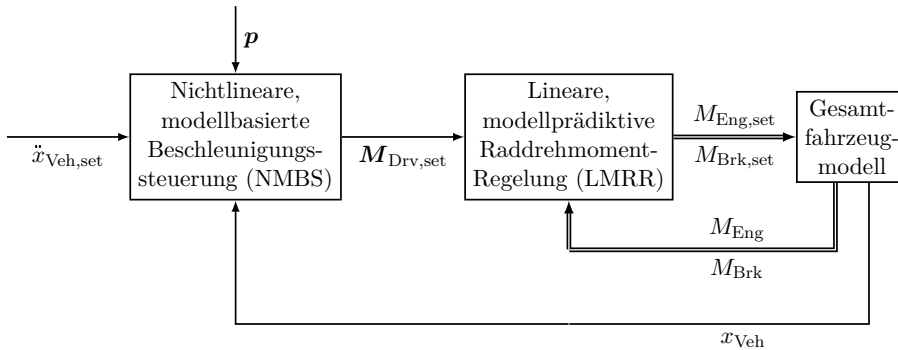
Abbildung 4.11: Signalflussdiagramm der Synthese von NMBS und LMRR.
