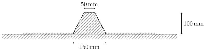
(e) Stopper mit einem trapezförmigen Querschnitt.
