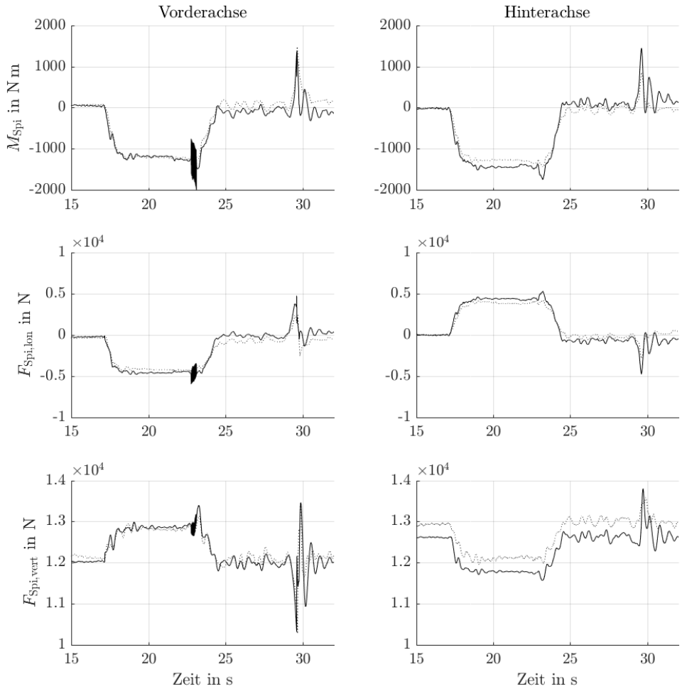
Abbildung C.4: Messung #676
