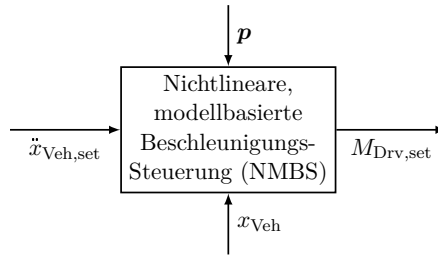
Abbildung 3.19: Eingänge und Ausgänge der NMBS.
