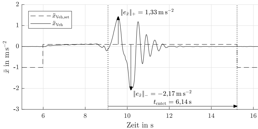
(a) Beschleunigungsverlauf
