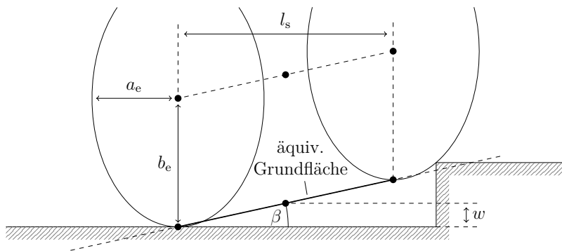
Abbildung 2.3: Das Tandemmodell elliptischer Kämme, mit denen das Fahrprofil abgetastet und daraus die äquivalente Grundfläche (fett) ermittelt wird.
