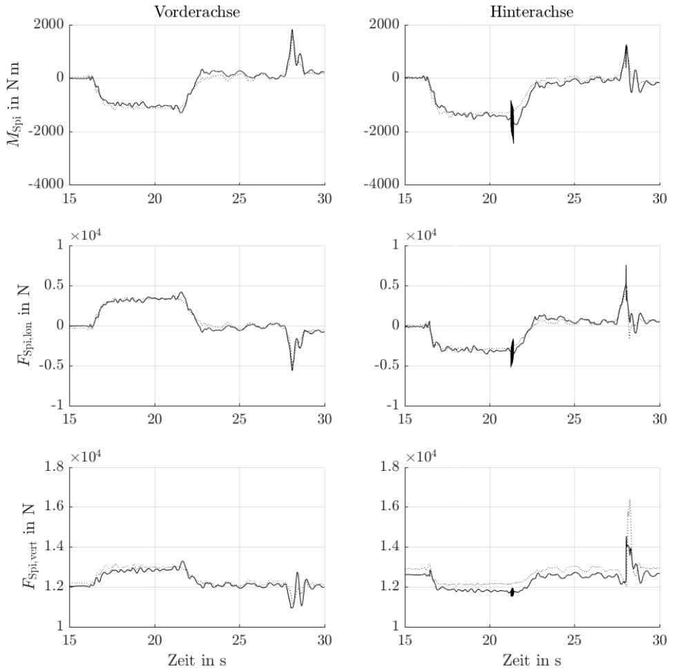
Abbildung C.6: Messung #700
