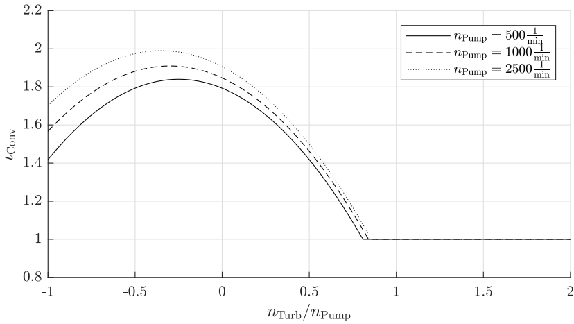
Abbildung A.2: Idealierte Wandlerkennlinien für verschiedene Pumpendrehzahlen.
