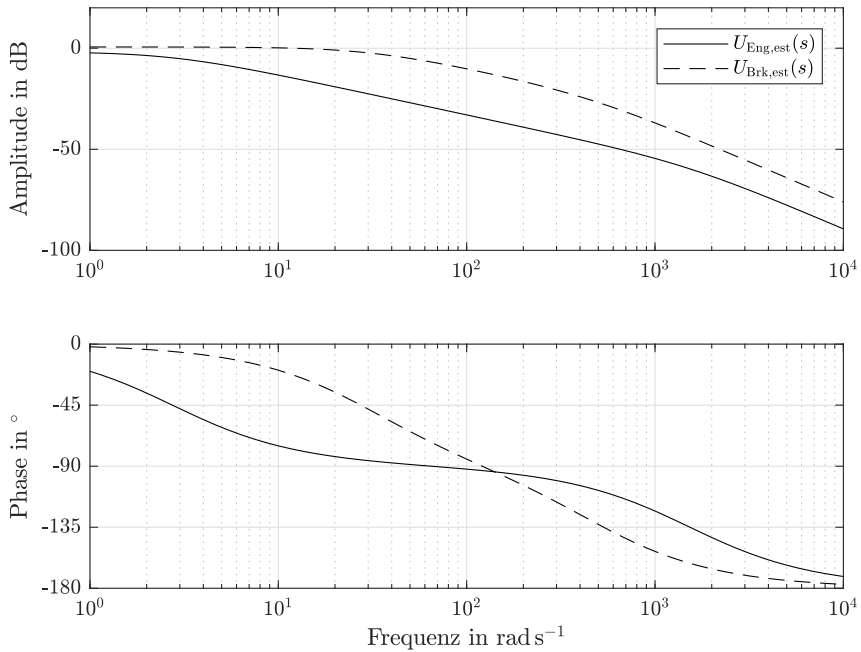
Abbildung C.21: Die Bodediagramme der identifizierten PT2-Modelle U_{Eng,est}(s) und U_{Brk,est}(s) .
