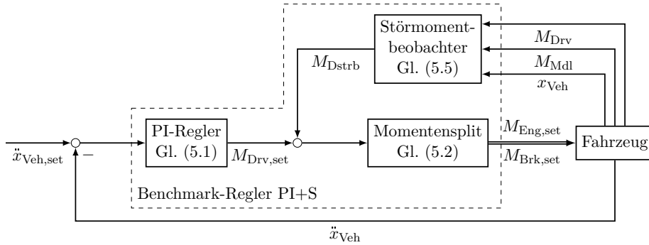
Abbildung 5.1: PI-Regler mit Störgrößenaufschaltung im geschlossenen Kreis wie er bei den in diesem Kapitel gezeigten Vergleichsmessungen zum Einsatz kommt.
