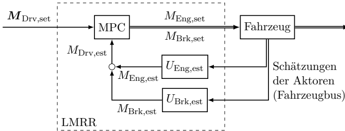
Abbildung 4.10: Signalflussdiagramm der LMRR.
