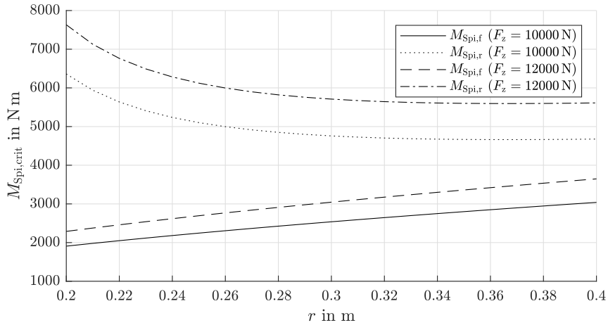
Abbildung A.5: Das erforderliche Drehmoment an den Rädern der angetriebenen Achse zum Anfahren vor einem stufenförmigen Hindernis mit einer Höhe von 14 cm in Abhängigkeit des Radius' des Rades r , wenn die starren Räder der Vorderachse genau am Hindernis stehen.
