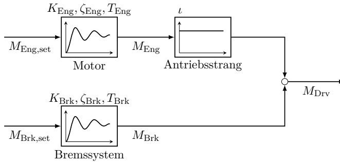
Abbildung 4.3: Signalfussdiagramm der Regelstrecke der LMRR.
