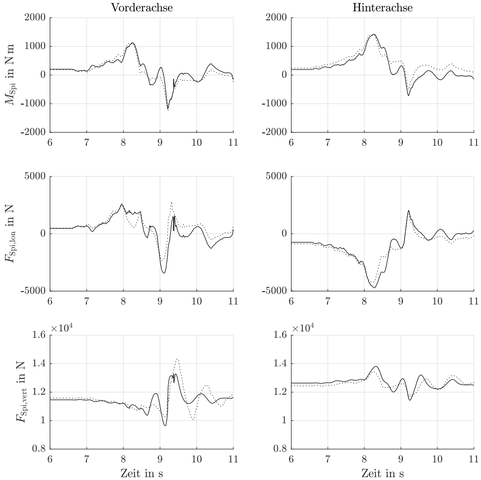
Abbildung C.7: Messung #830
