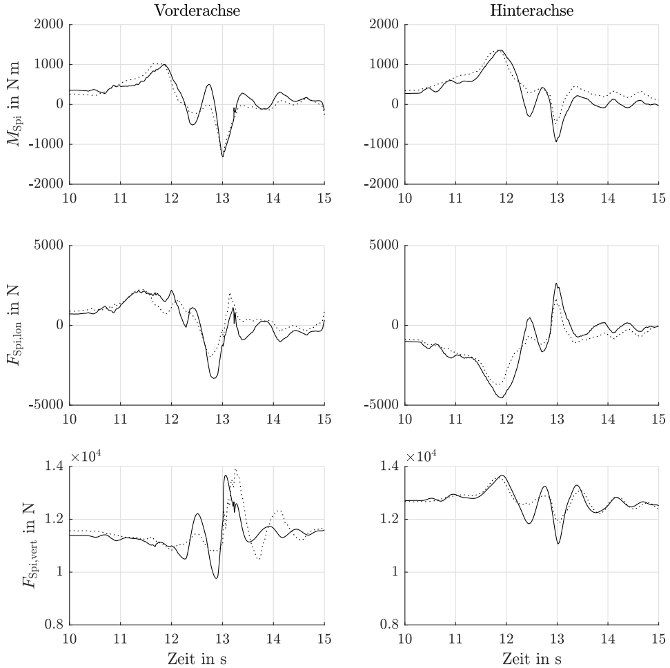
Abbildung C.9: Messung #742
