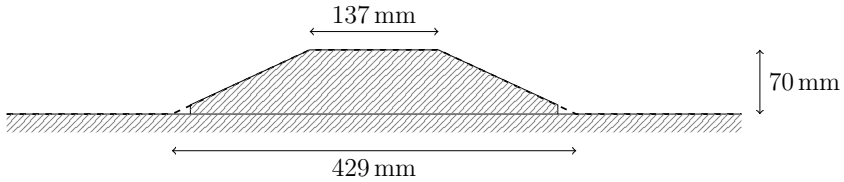
(c) Kabelbrücke mit einem trapezförmigen Querschnitt.
