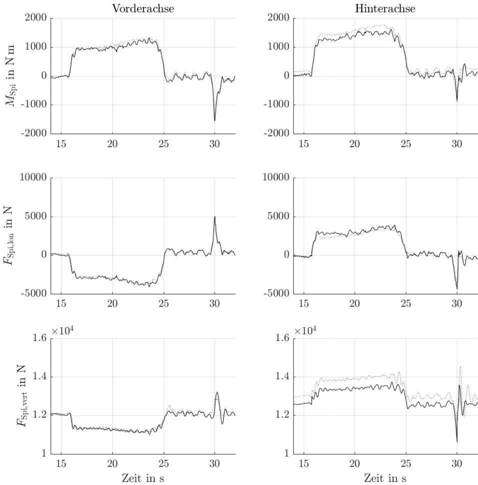
Abbildung C.5: Messung #701
