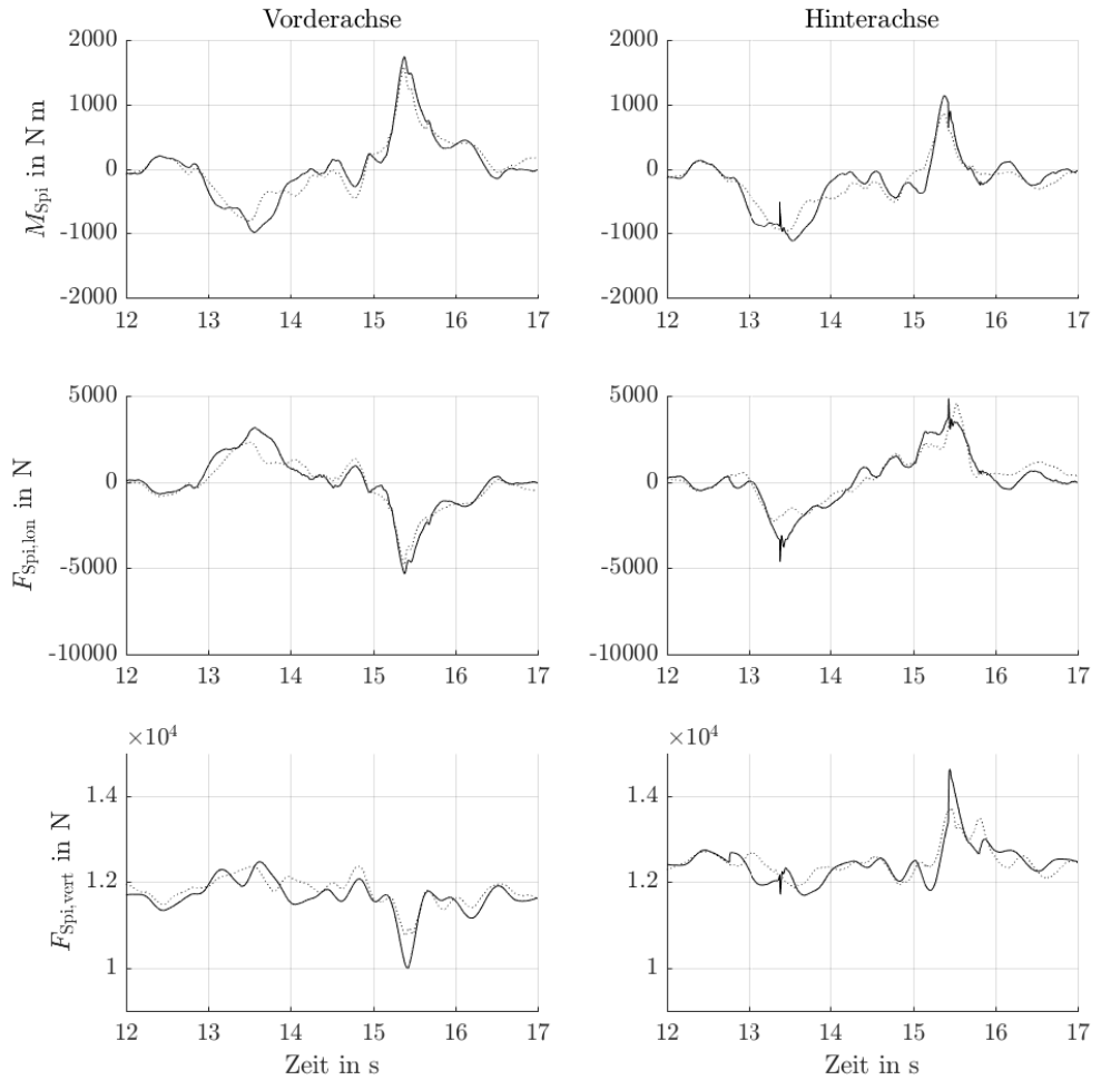
Abbildung C.8: Messung #875
