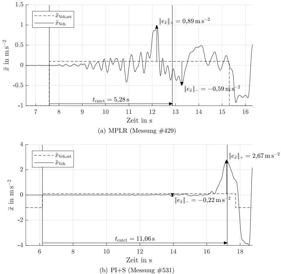
Abbildung 5.7: Beispielhafte Ergebnisse für das Anfahren vor einer 14 cm hohen Stufe mit MPLR und PI+S.
