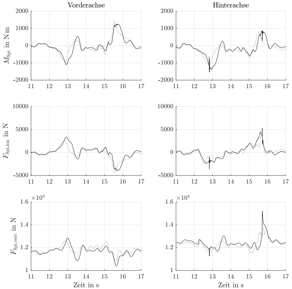
Abbildung C.10: Messung #789
