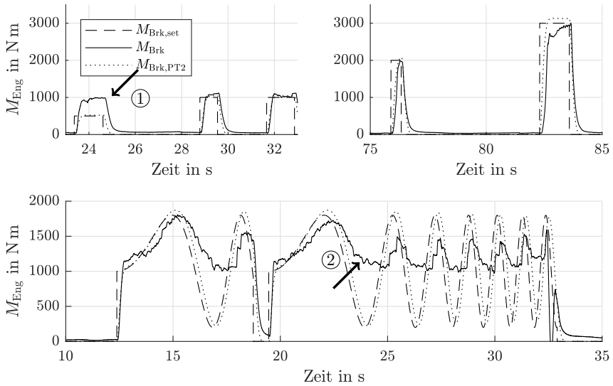
Abbildung 4.7: Messungen mit Sollwertsprüngen (oben) und einem Chirp-Signal (unten) zur Identifizierung der Übertragungsfunktion U_{Brk}(s) des Bremssystems im schnellen Modus.
