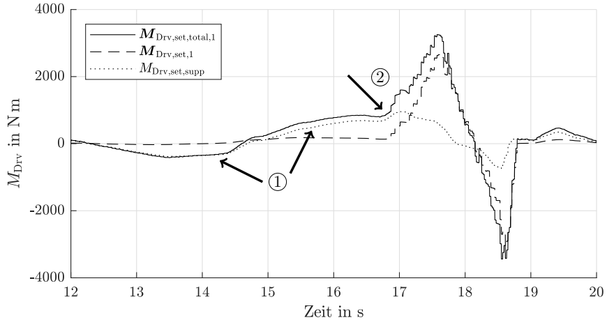
Abbildung 5.3: Beispielhafter Verlauf des ersten Elements von \mathbf{M}_{\text{Drv, set, total}} (durchgezogener Graph) sowie der von NMBS (gestrichelt) und SKR (gepunktet) geforderten Drehmomente beim Überfahren des Stoppers.
