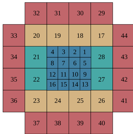
■ T2 trigger, ■ + ■ + ■ 30A, 40A and 75A, ■ + ■ + ■ + ■ 13A and 19A GeV/c.
