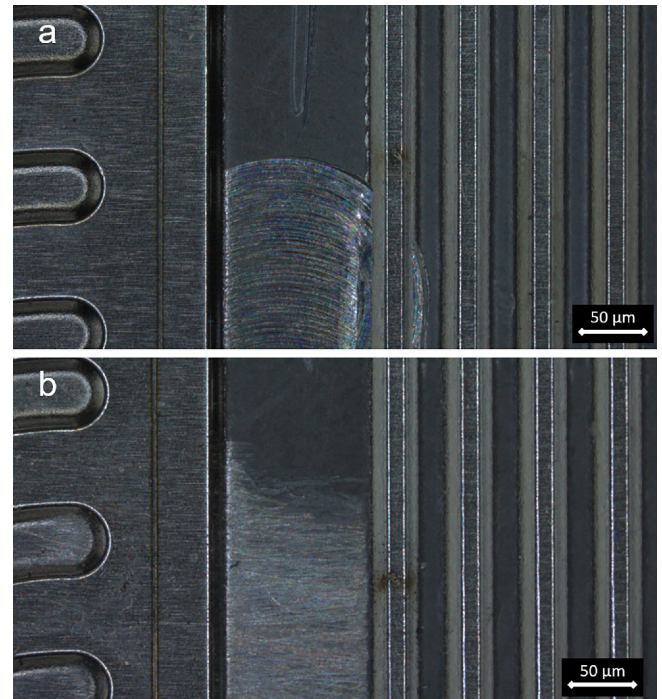
Bild 5. Versuche zur Defekteinbringung in die Beschichtung (a: Fräsmaschine, b: manuell Schmirgelpapier). Foto: wbk, Karlsruher Institut für Technologie
