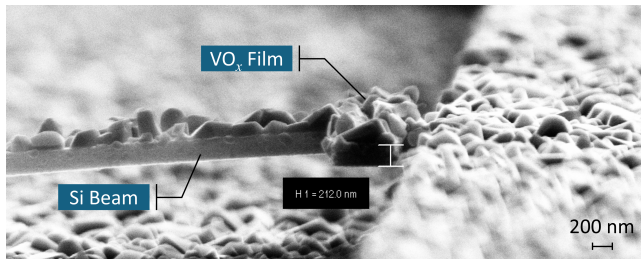
(b) VO x film
