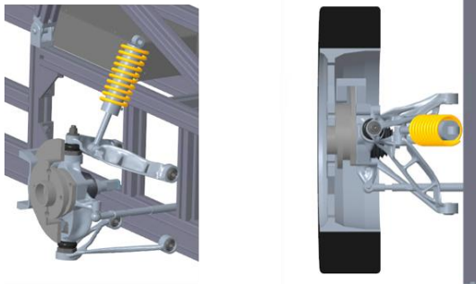
Abbildung B-44: Gesamtsystem der Vorderachse der Fahrzeugkonfiguration Cargo, links: Seitenansicht, rechts: Draufsicht [Haw-24]
