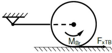
Abbildung 2-18: Längslenkerradaufhängung [Gie-23]
