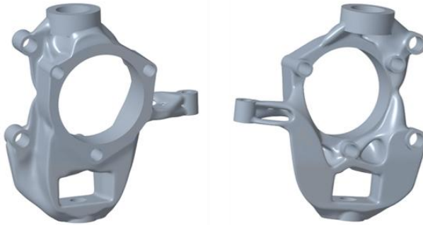
Abbildung 4-36: Finales CAD-Modell des Radträgers, links: radseitige Ansicht, rechts: aufbauseitige Ansicht [Haw-24]
