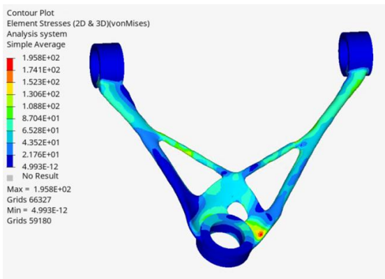
Abbildung B-33: FEM -Analyse des oberen Querlenkers der Fahrzeugkonfiguration Track, Lastfall Längsstoß [Haw-24]
