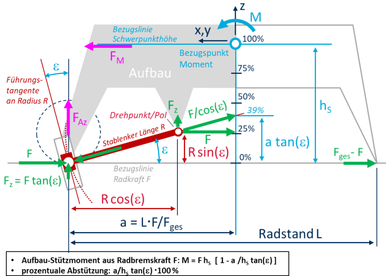
Abbildung 2-9: Aufbaustützung aufgrund Bremsstützwinkel \epsilon aus Radstandänderung über Einfederung bei Bremsmomentenabstüzung am Radträger [Sch-24]
