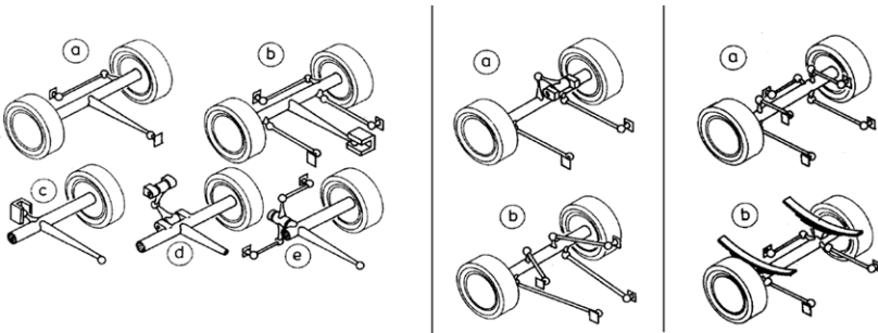
Abbildung 2-12: Übersicht möglicher Starrachsenausführungen (Quelle Bilder: [Mat-07])
