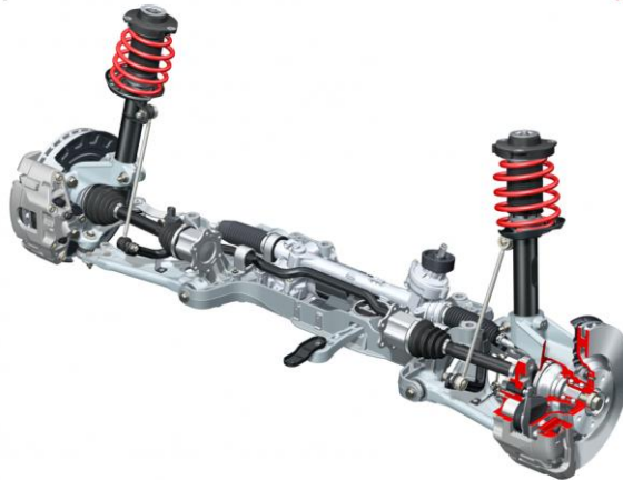
Abbildung 2-17: Ausgeführte McPherson-Radaufhängung an der Vorderachse eines Audi TT [Aud-25]
