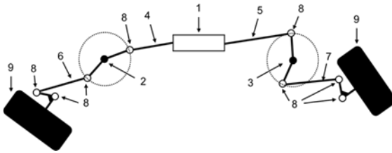
Abbildung 4-8: Lenkgestänge bei Kurvenfahrt [Wei-24-4]
