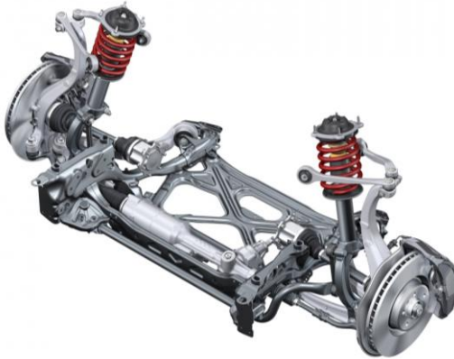
Abbildung 2-27: Ausgeführte Mehrlenkerradaufhängung am Beispiel einer Fünflenker-Vorderachse des Audi A6 [Aud-25]
