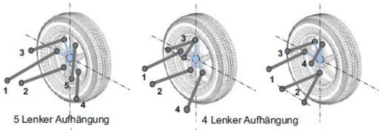
Abbildung 2-26: Mehlenkerradaufhängungen [Ers-17d]
