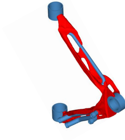
Abbildung 4-21: Ergebnis der Topologieoptimierung des oberen Querlenkers, rot: genutzter Designspace, blau: Non-Designspace [Wei-24-6]
