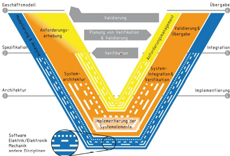
Abbildung 2-33: V-Modell [VDI-21]
