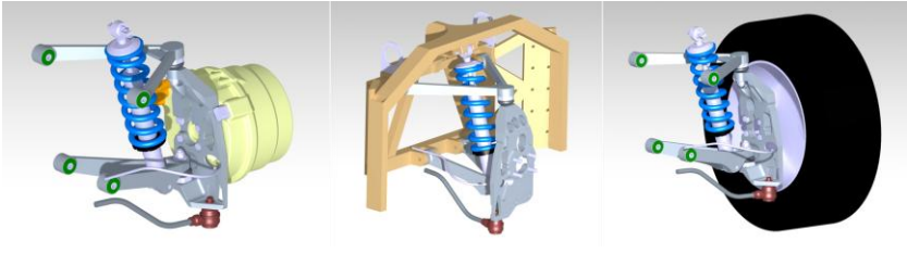
Abbildung 4-22: Gesamtmodell der Vorderachse mit links: Spurstange und Radnabenmotor, Mitte: Spurstange und Fahrschemel, rechts: Spurstange und Rad
