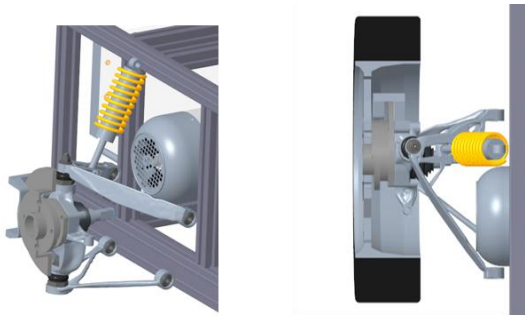
Abbildung B-45: Gesamtsystem der Hinterachse der Fahrzeugkonfiguration Cargo, links: Seitenansicht, rechts: Draufsicht [Haw-24]
