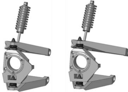
Abbildung B-15: Designspace der Radaufhängung der Fahrzeugkonfiguration Cargo, links: Vorderachse, rechts: Hinterachse [Haw-24]
