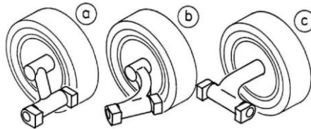
Abbildung 2-22: Vergleich: a Längslenker, b Schräglenker, c Pendelachse [Gie-23]
