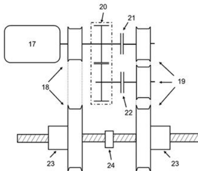
Abbildung 4-9: Lenkgetriebe bei Geradeausfahrt [Wei-24-4]
