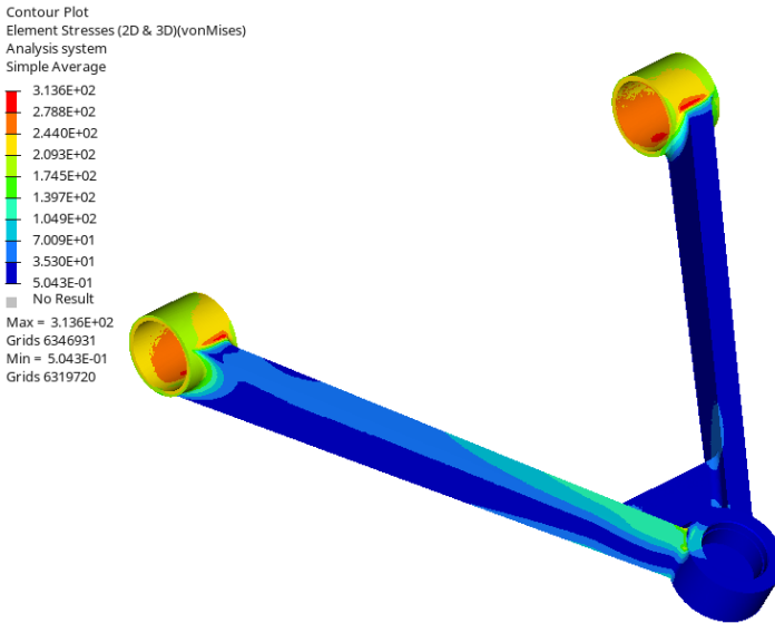
Abbildung 4-19: FEM-Analyse des oberen Querlenkers, Lastfall Längsstoß
