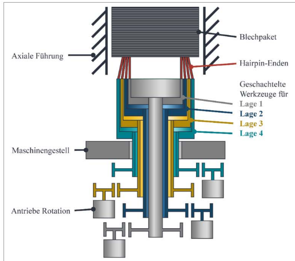
Bild 3 Schematischer Aufbau einer simultanen Twistanlage mit konzentrisch geschachtelten Twistwerkzeugen, hier mit axialer Zustellung des Stators. Grafik: wbk
