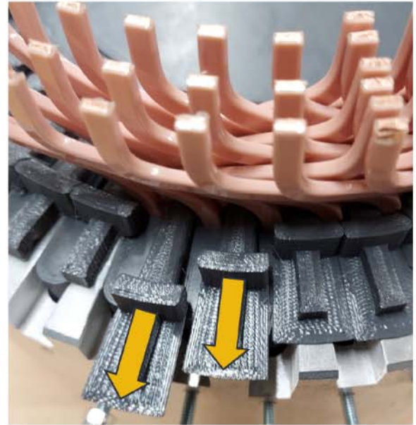
Bild 6 Additiv gefertigter Stützfingerring zum Schutz aller Drähte eines Hairpin-Stators während des Twistprozesses. Links: Stützfinger mit eingesetztem Keil, Rechts: Entnahme der Stützfinger. Grafik: wbk
