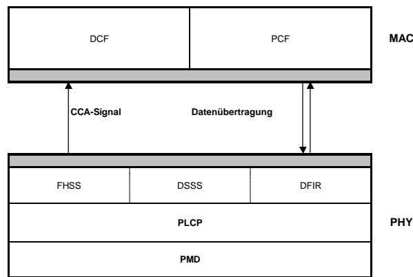
Abbildung 3: 802.11-Protokollarchitektur
