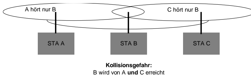
Abbildung 11: Versteckte Endgeräte
