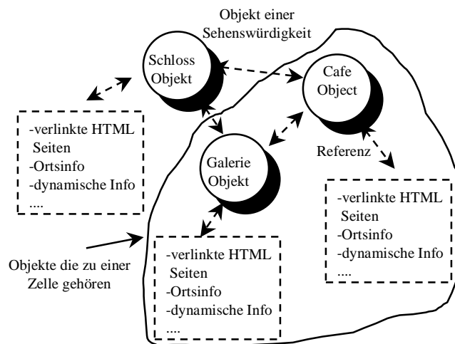
Abbildung 5: Objektmodell
