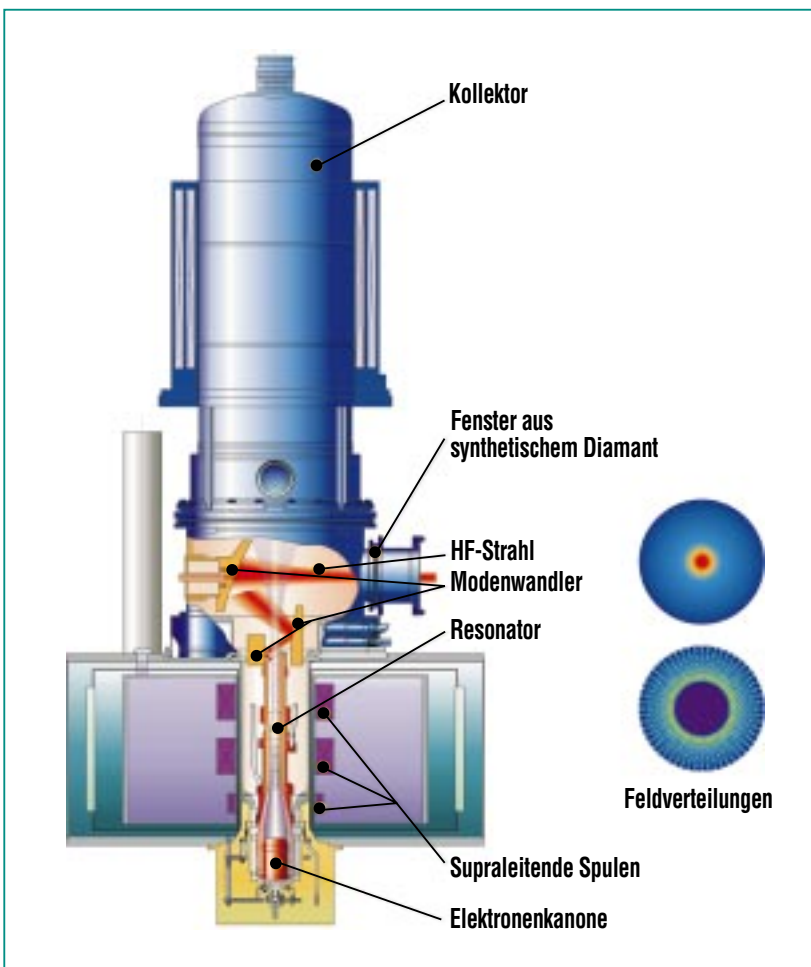
Abb. 1: Schematischer Aufbau eines Gyrotrons mit der Elektronenkanone, dem supraleitenden Magnetsystem, dem Resonator, dem Modenwandler, dem Diamantfenster und dem Kollektor. Auf der rechten Seite ist die Feldverteilung am Auskoppelfenster (oben) und im Resonator (unten) dargestellt. Die Umwandlung geschieht mittels eines optimierten Modenwandlers.
