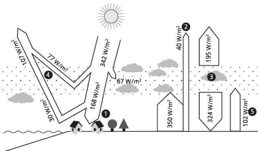
ABB. III.3 SCHEMATISCHE DARSTELLUNG DER STRAHLUNGSBILANZ DER ERDE
