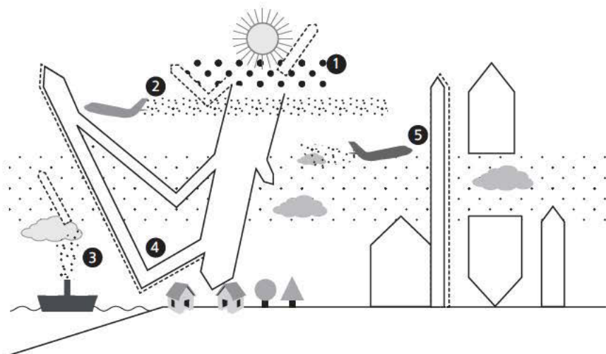
ABB. III.4 DISKUTIERTÉ MÖGLICHKEITEN ZUR TECHNISCHEN BEEINFLUSSUNG DER STRAHLUNGSBILANZ DER ERDE
