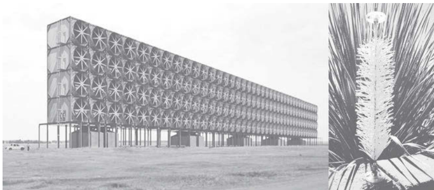
ANLAGENKONZEPTE ZUR \text{CO}_2 -ABSCHEIDUNG AUS DER LUFT
