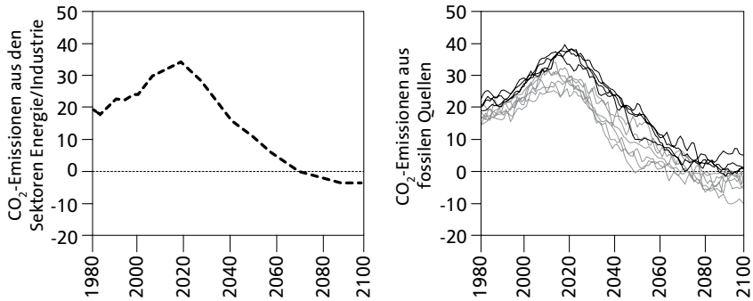
ABB. VI.2 MIT DEM SZENARIO RCP2.6 KOMPATIBLE \text{CO}_2 -EMISSIONSPFADE ANHAND VERSCHIEDENER MODELLIERUNGEN (IN MRD. \text{t CO}_2/\text{JAHR} )
