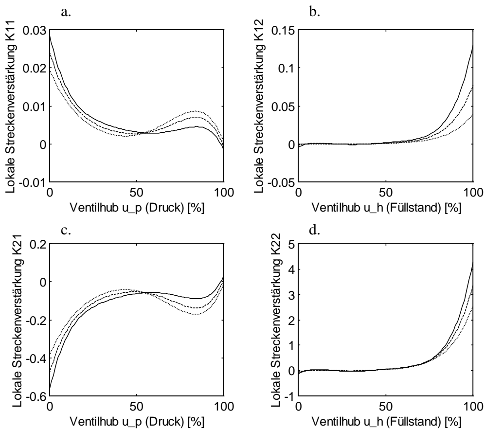
Bild 4.9: Lokal gültige Streckenverstärkungen Hauptstrecke Druck \partial f_{11}(u_{p,p})/\partial u_p (oben links) Koppelstrecke Füllstand \rightarrow Druck \partial f_{12}(u_{h,p})/\partial u_h (oben rechts) Koppelstrecke Druck \rightarrow Füllstand \partial f_{21}(u_{p,p})/\partial u_p (unten links) Hauptstrecke Füllstand \partial f_{22}(u_{h,p})/\partial u_h (unten rechts)
