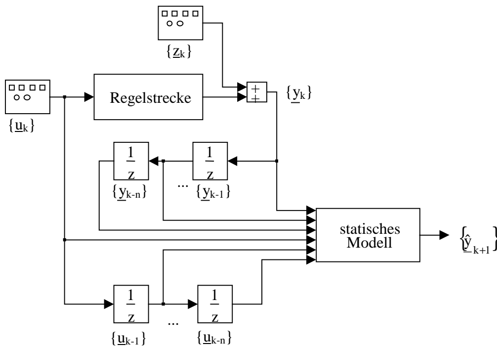
Bild 3.13: Seriell-paralleles Modell
