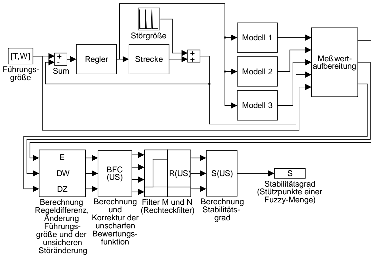
Bild 3.24: MATLAB-Struktur mit Regelkreis, Modellen mit unsicheren Parametern und Überwachungsebene
