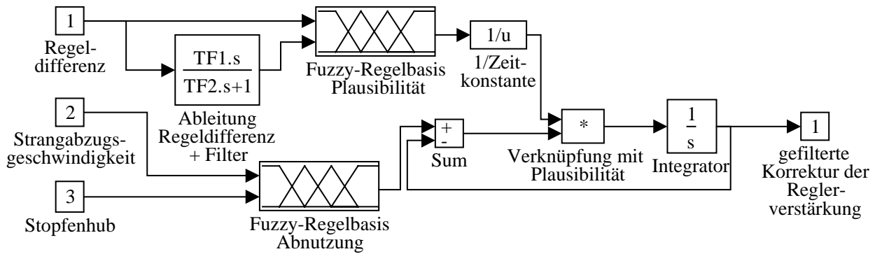
Bild 4.18: MATLAB-Struktur des Fuzzy-Blocks zur Ermittlung der Reglerverstärkung
