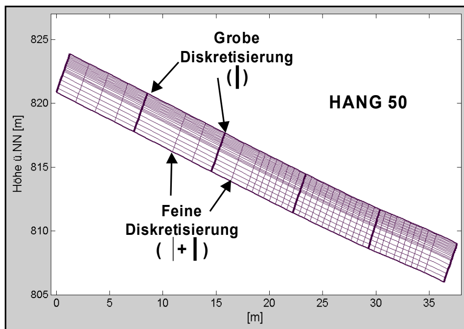
Abbildung 5-22: Zwei Diskretisierungsvarianten für den Hang 50
