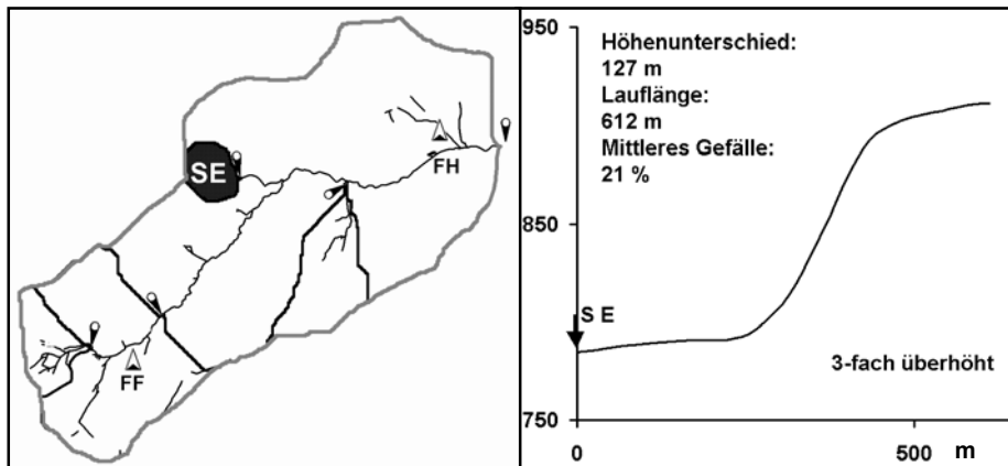
Abbildung 4-21: Lage und Längsprofil des Einzugsgebietes SE
