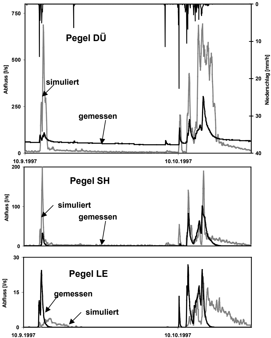
Abbildung 5-19: CATFLOW: Zwei Beispiereignisse an den Pegel DÜ, SH und LE
