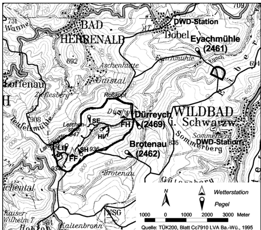
Abbildung 2-2: Lage des Einzugsgebietes, Nachbarpegel
