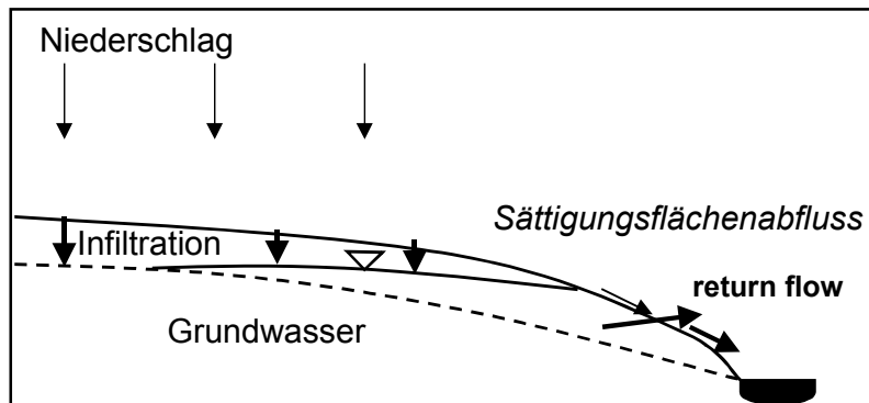
Abbildung 2-13: Sättigungsflächenabfluss („Saturation Excess Flow“)
