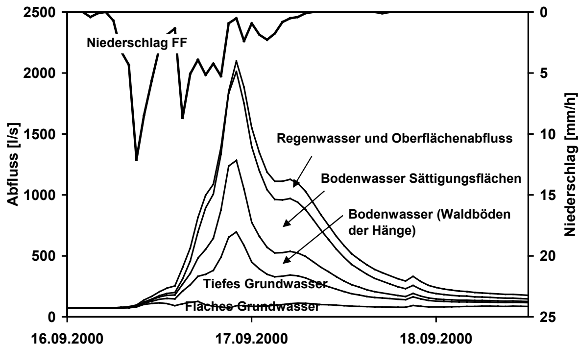
Abbildung 4-35: Trennung in 5 Abflusskomponenten am Pegel DÜ
