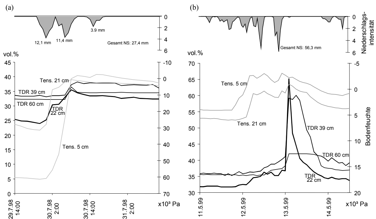
Abbildung 6: Tiefenausbreitung von Bodenwasser am Bodenprofil 2 (P2) nach Niederschlagsereignissen bei (a) trockenen und (b) feuchten Vorbedingungen.
