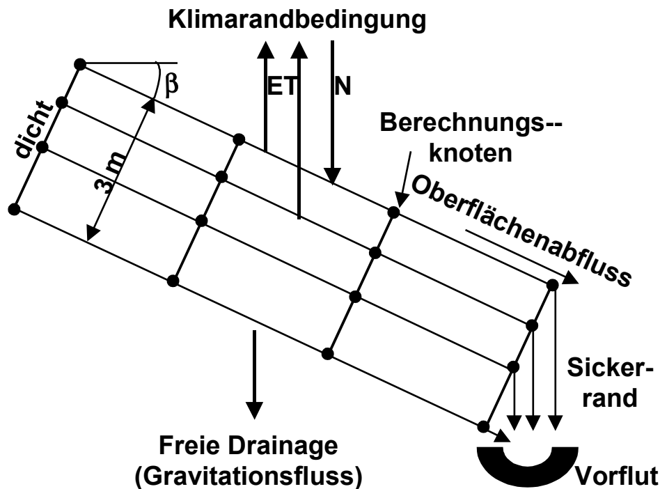
Abbildung 5-17: CATFLOW: Flussrandbedingungen an einem Hangsegment (schematisch)
