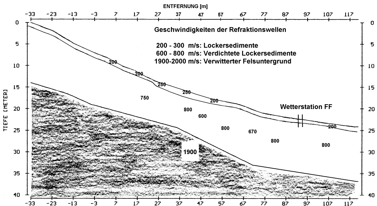
Abbildung 4-11 : Geophysikalisches Profil bei FF (aus FLINSPACH, 1999, verändert)
