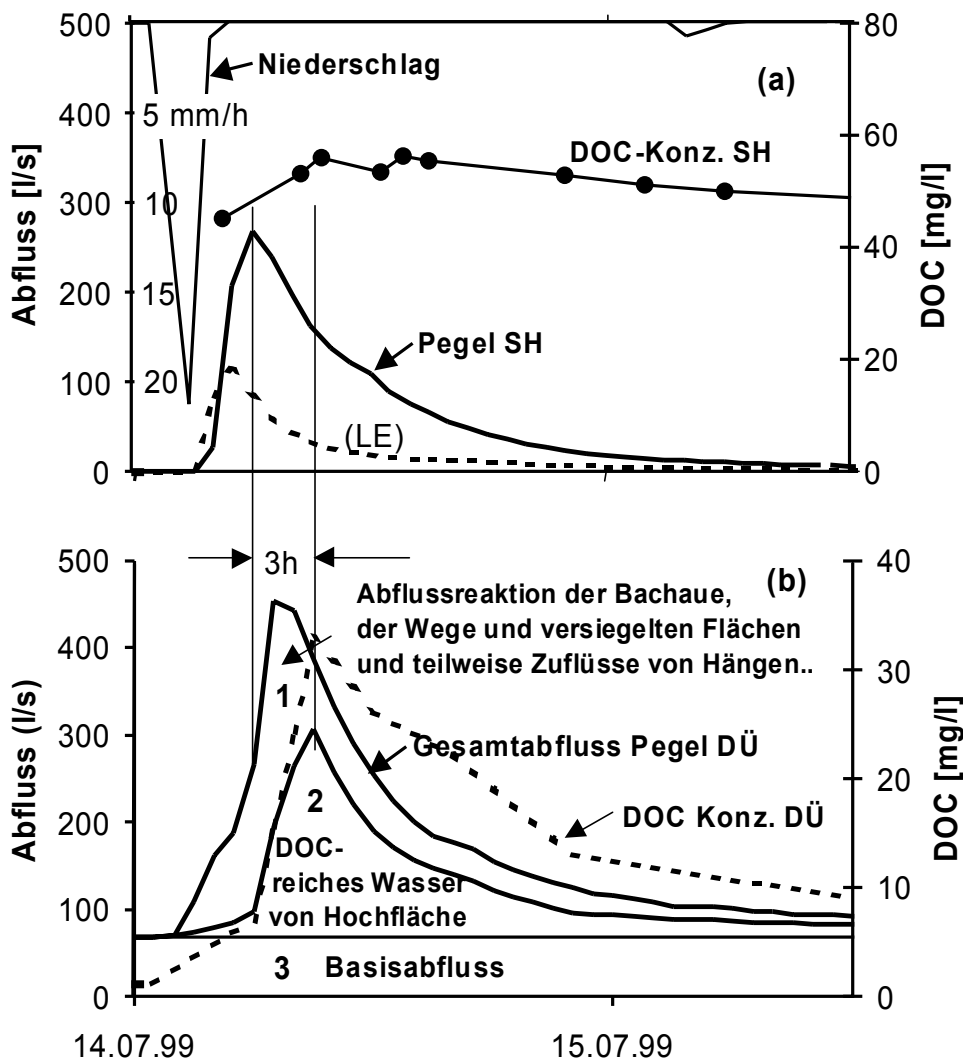
Abbildung 4-23: Komponententrennung am Hauptpegel über DOC-Bilanzierung
