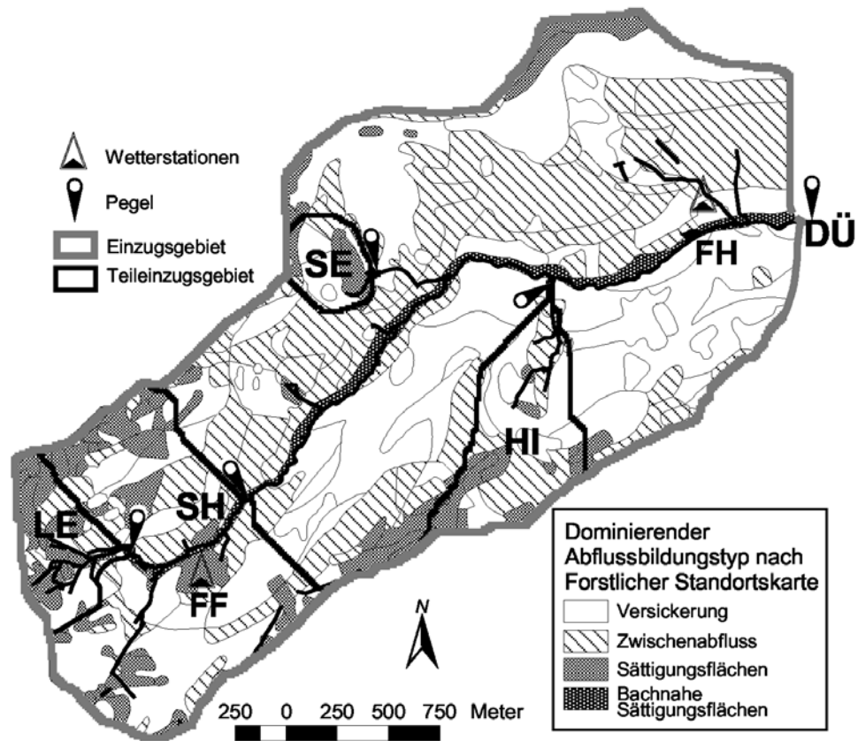
Abbildung 4-14: Dominierender Abflussbildungstyp (WALDENMEYER, 1999)
