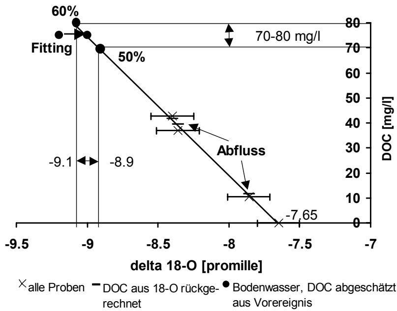
Abbildung 4-17: Messungen für DOC und \delta^{18}\text{O} am Pegel LE (4./5.8.1999)
