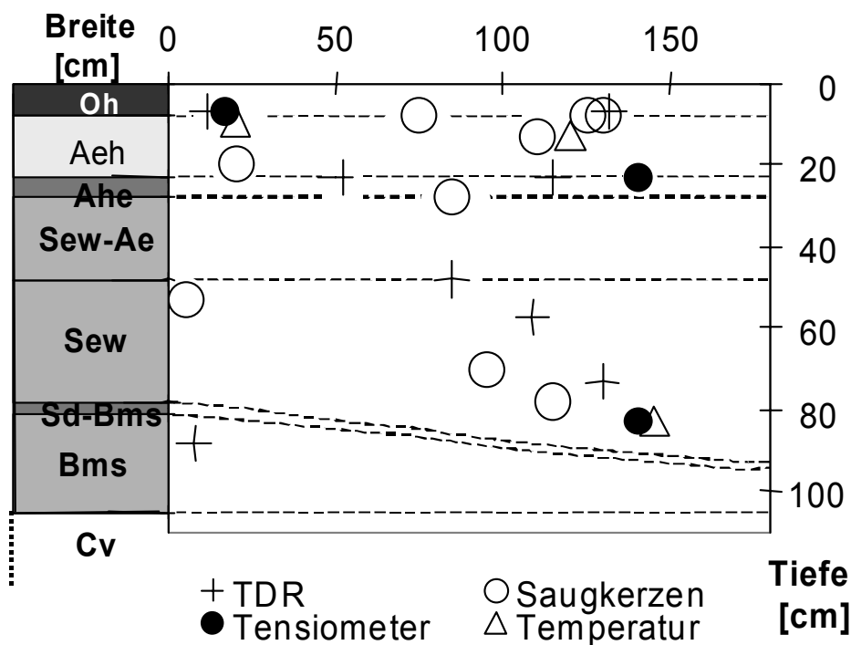
Abbildung 1: Bodenprofil 1 (P 1): Profilaufbau und Lage der Messeinrichtungen
