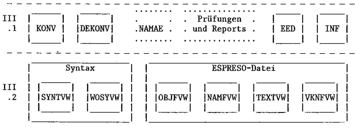
Bild 4.2 Struktur der Schicht III
