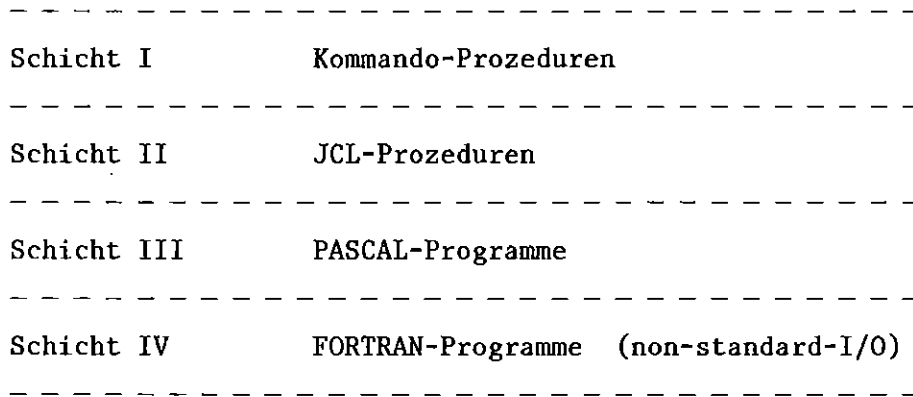
Bild 4.1 Schichtenstruktur von ESPRESO-W
