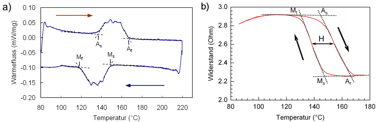
Abbildung 4.2: a) DSC-Messung und b) Widerstand-Temperatur-Kennlinie eines \text{Ni}_2\text{MnGa}_{50\text{W}} -Dünnsfilms.
