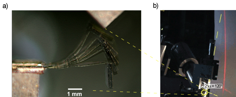
Abbildung 5.10: Dynamischer Betrieb eines Spiegelaktors mit Design 1 in einer Langzeitbelichtung a) und unter dem Winkel 2\Delta\alpha von 120^\circ abgelenkter Laserstrahl, der die Form einer geraden Linie beschreibt b).
