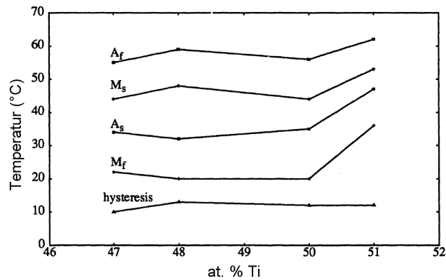
Abbildung 2.11: Umwandlungstemperaturen von NiTiCu-Legierungen und Breite der Hysterese in Abhängigkeit vom Ti-Gehalt [22].
