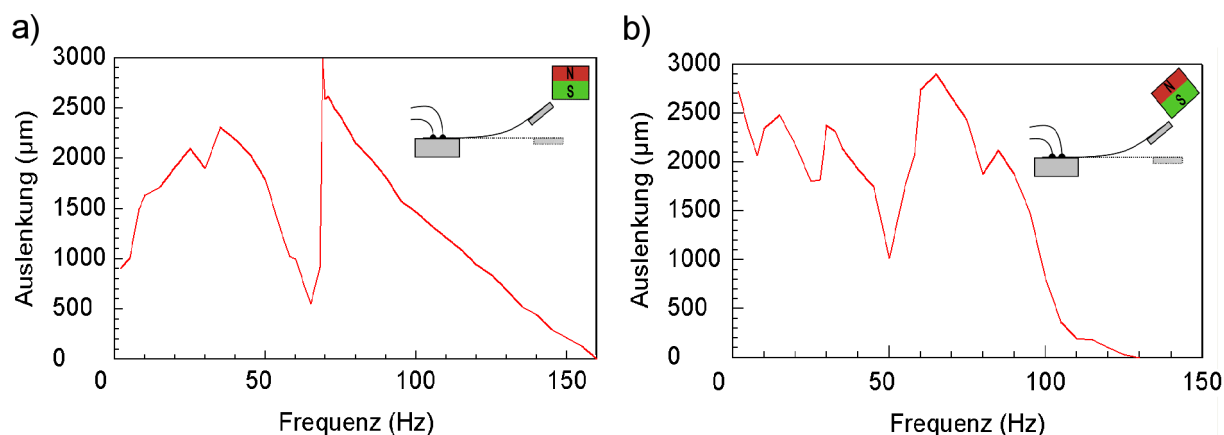
Abbildung 5.11: Auslenkung-Frequenz-Kennlinie eines Spiegelaktors mit Design 1 für einen Drehwinkel von 0^\circ a) und 45^\circ b).
