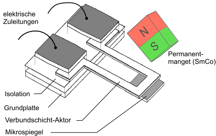
Abbildung 5.38: Schematischer Aufbau des Spiegelaktors basierend auf einer Verbundschicht mit weichmagnetischen Material.
