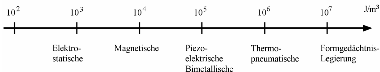
Abbildung 2.1: Energiedichte verschiedener Aktorprinzipien [6].
