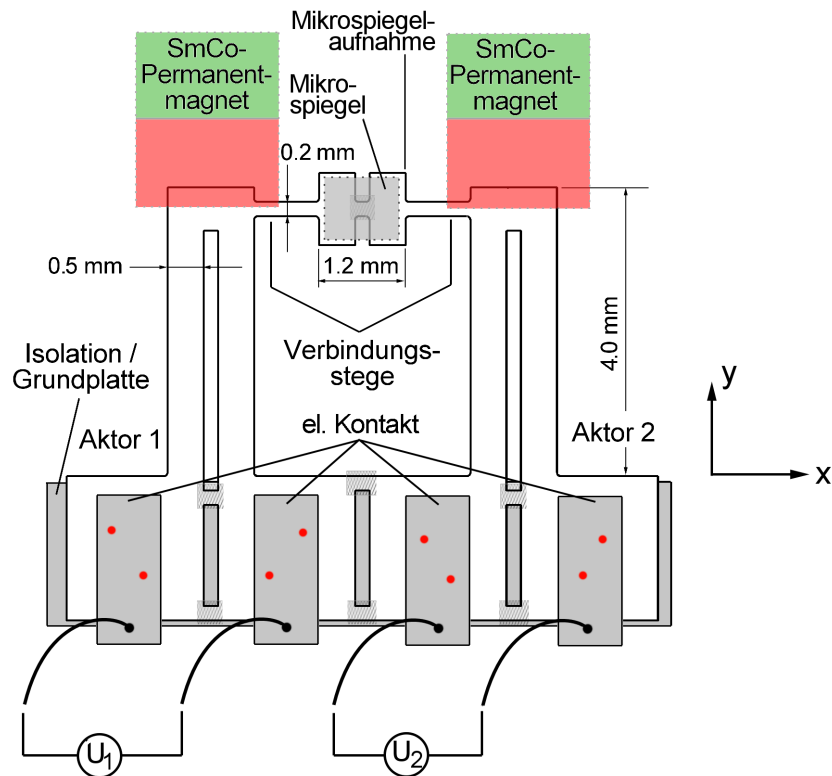
Abbildung 6.1: Schematisch dargestelltes Design des ferromagnetischen \text{Ni}_2\text{MnGa} -Spiegelaktors zur zweidimensionalen Strahlableitung in Draufsicht.
