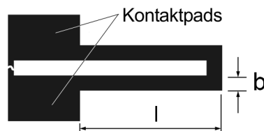
Abbildung 3.5: Design der Doppelbiegebalken-Teststruktur.
