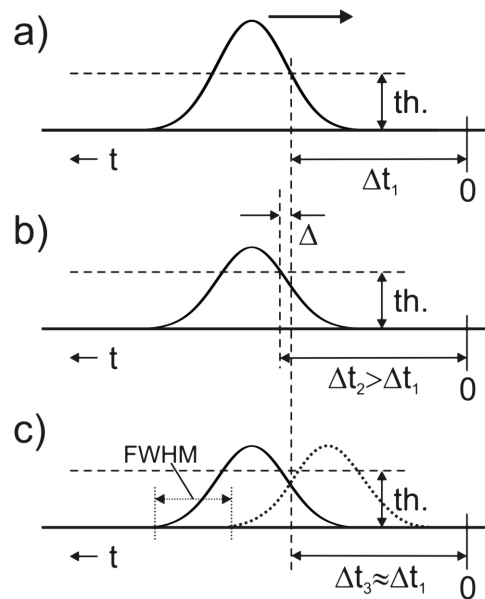
Abbildung 7.6: Prinzip des Schwellwertdetektors; a) mit fester Schwelle, b) bei kleinem Puls und c) CFD bei kleinem Puls [52]. Legende: th. = threshold , Schwellwert; \Delta = zeitliche Messabweichung; \Delta t_{1,2,3} = ermittelte Messwerte.
