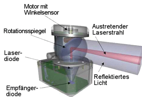
Abbildung 7.1: Funktionsprinzip des Alasca® Laserscanners der IBEO AS GmbH [51].
