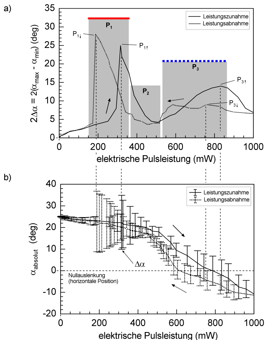
Abbildung 5.15: Scanwinkel–Leistungs–Kennlinie a) und absoluter Winkel \alpha_{\text{absolut}} für eine Pulsfrequenz von 76.0 Hz b). Die Balken geben die maximale und minimale Auslenkung des Scanners an, aus der die Scanamplitude 2\Delta\alpha resultiert.
