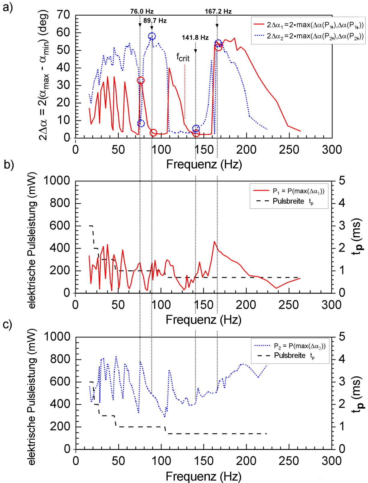
Abbildung 5.14: Scanwinkel–Frequenz–Kennlinie eines Spiegelaktors mit Design 2 in Abhängigkeit von der elektrischen Pulsleistung und der Pulsdauer t_p .
