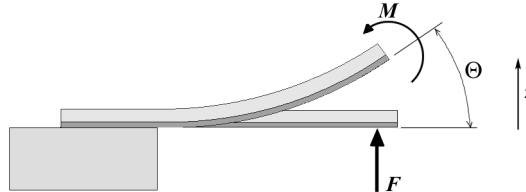
Abbildung 2.4: Schematische Darstellung der Auslenkung einer Verbundschicht.
