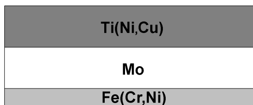
Abbildung 3.1: Schichtverbund mit NiTiCu FGL–Verbundschicht.
