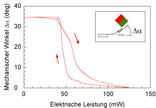
Abbildung 5.7: Auslenkung–Leistung–Kennlinie eines Spiegelaktors mit Abmessungen nach Design 1.
