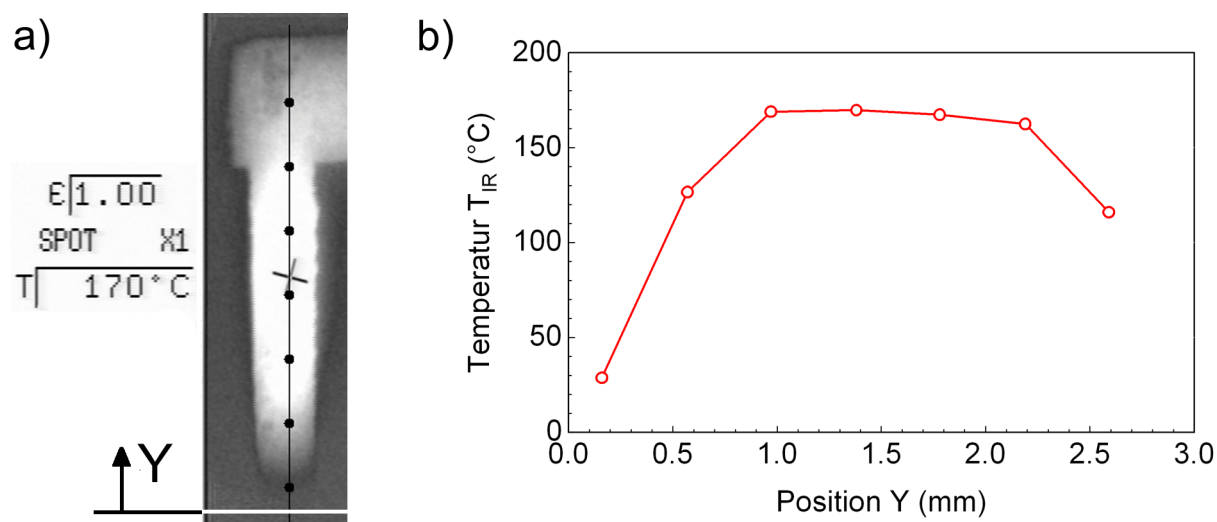
Abbildung 4.5: a) IR-Graustufenbild eines Steges des Doppelbiegebalkens und b) entlang der Mittellinie des Steges in y-Richtung ermittelte Temperaturen.
