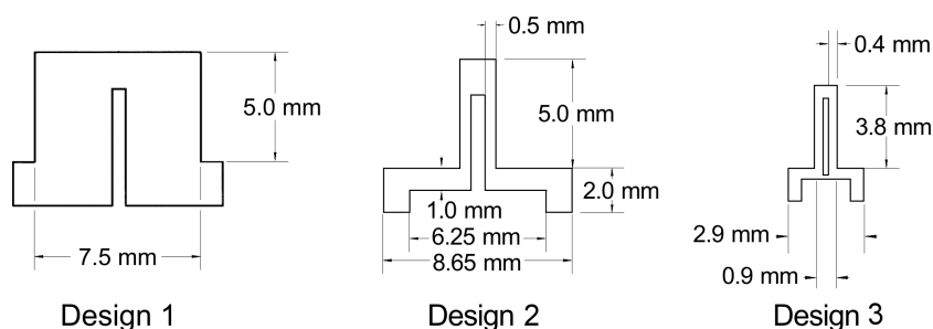
Abbildung 5.28: Designs der NiTiCu-Verbundschichtaktoren.
