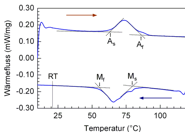
Abbildung 4.3: DSC-Messung eines \text{Ni}_2\text{MnGa}_{200\text{W}} -Dünnsfilms.
