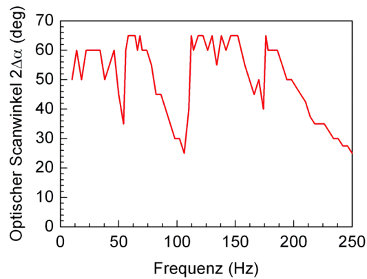
Abbildung 5.22: Scanwinkel–Frequenz–Kennlinie für einen Ni_2MnGa -Aktor mit Design 2.
