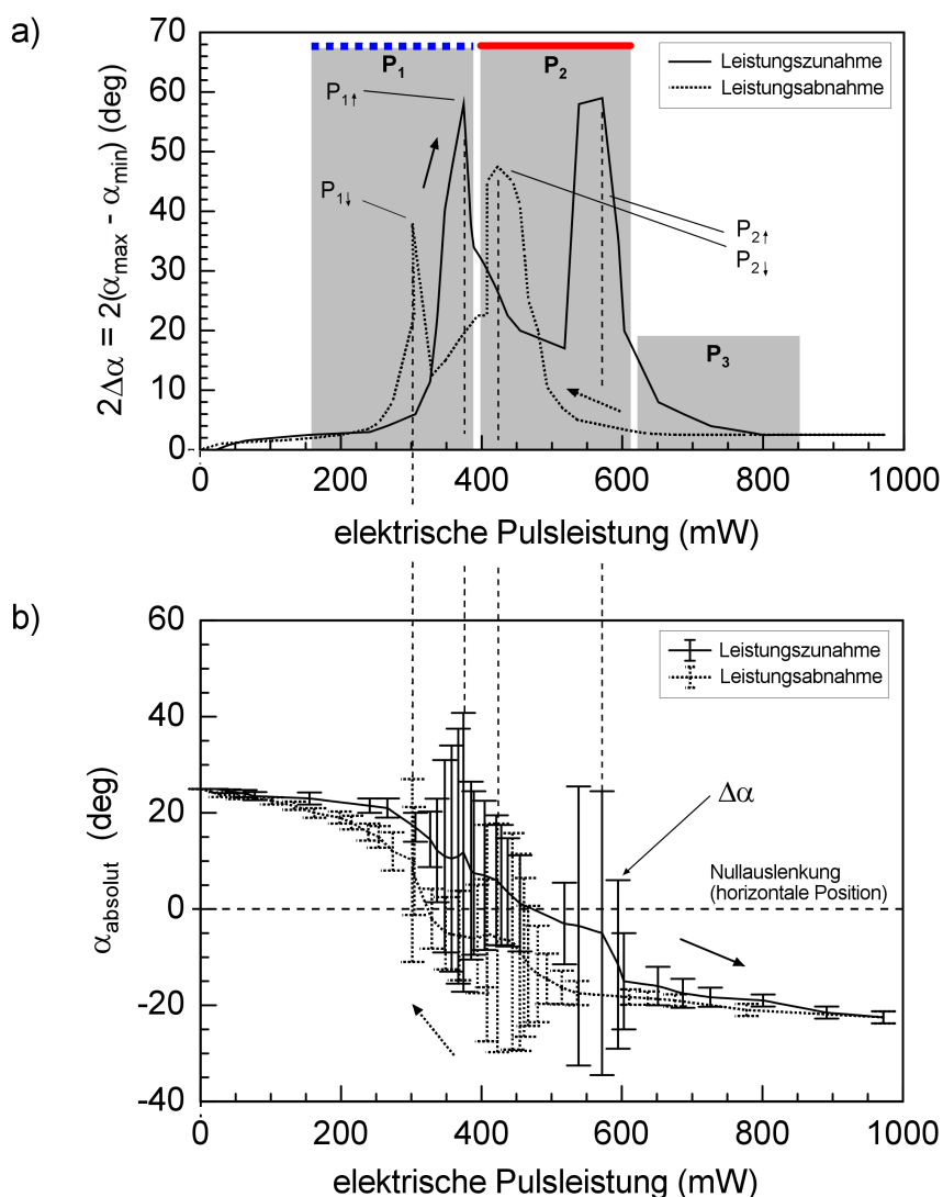
Abbildung 5.18: Scanwinkel–Leistungs–Kennlinie und absoluter Winkel \alpha_{\text{absolut}} für eine Pulsfrequenz von 167.2 Hz.
