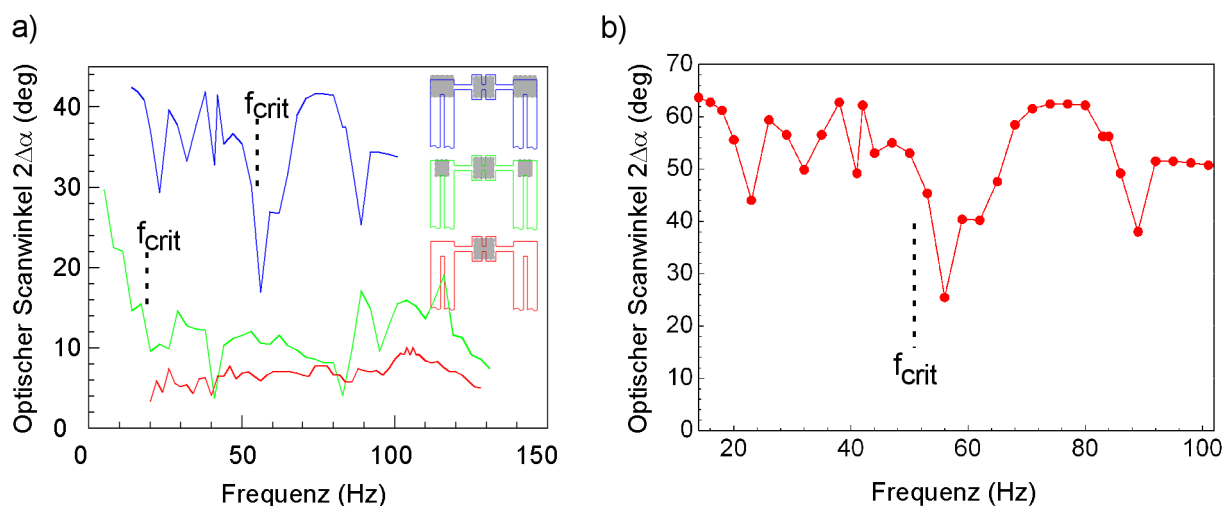
Abbildung 6.5: Scanwinkel–Frequenz–Kennlinien a) in Abhängigkeit unterschiedlicher Massen am vorderen Ende der frei beweglichen Doppelbiegebalken–Strukturen für jeweils optimierte Pulsleistungen. In b) sind die Massen der verwendeten Mikrospiegel an den Doppelbiegebalken durch in der Form angepasste Cu–Gewichte gleicher Masse ersetzt.
