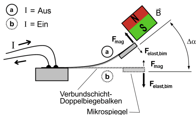
Abbildung 5.37: Funktionsprinzip des magnetischen Verbundschichtaktors aus FeCoBSi und Mo in der Seitenansicht. Legende: \vec{B} = Magnetfeld, I = elektrischer Strom, F_{mag} = magnetische Kraft, F_{elast,bim} = Rückstellkraft mit elastischem Anteil und Bimetall-Effekt, \Delta\alpha = mechanischer Ablenkwinkel.
