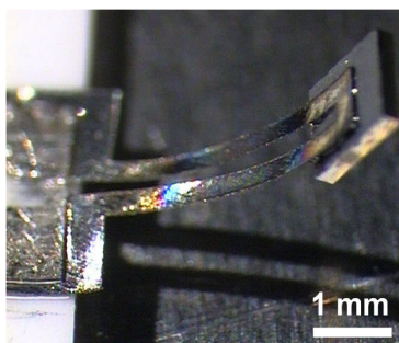
Abbildung 5.30: Prototyp eines Spiegelaktors bestehend aus einer NiTiCu-Verbundschicht mit Design 2 und Verbundschichtdicke a von 5.5 \mu\text{m} .
