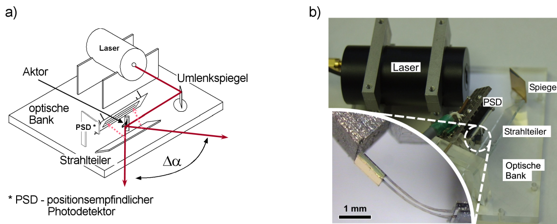
Abbildung 5.13: a) Schematischer Aufbau des Laserscanner-Demonstrators mit integrierter hochaufgelöster Winkelmessung und b) aufgebauter Demonstrator. Die Position des im Inset abgebildeten Spiegelaktors ist gekennzeichnet.
