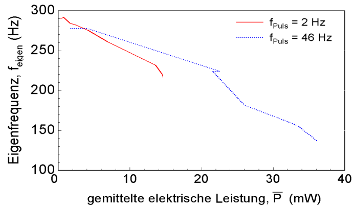
Abbildung 5.21: Berechnete Eigenfrequenz f_{eigen} für eine Anregung von 2 Hz und 46 Hz für unterschiedliche Pulsleistungen. In der Kennlinie dargestellt ist die gemittelte Leistung \bar{P} .
