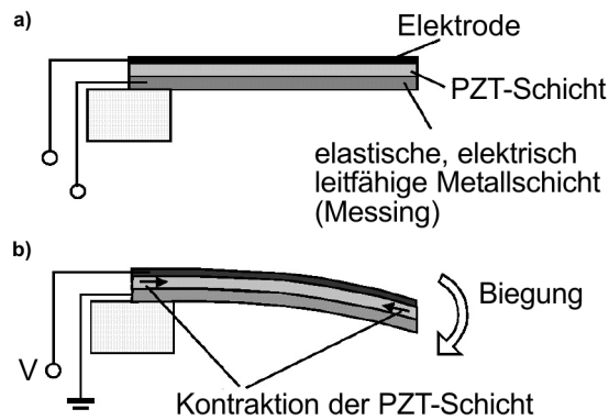
Abbildung 2.5: Schematischer Schichtaufbau a) und Funktionsprinzip b) eines unimorphen Biegebalken aus einlagigem PZT [15].
