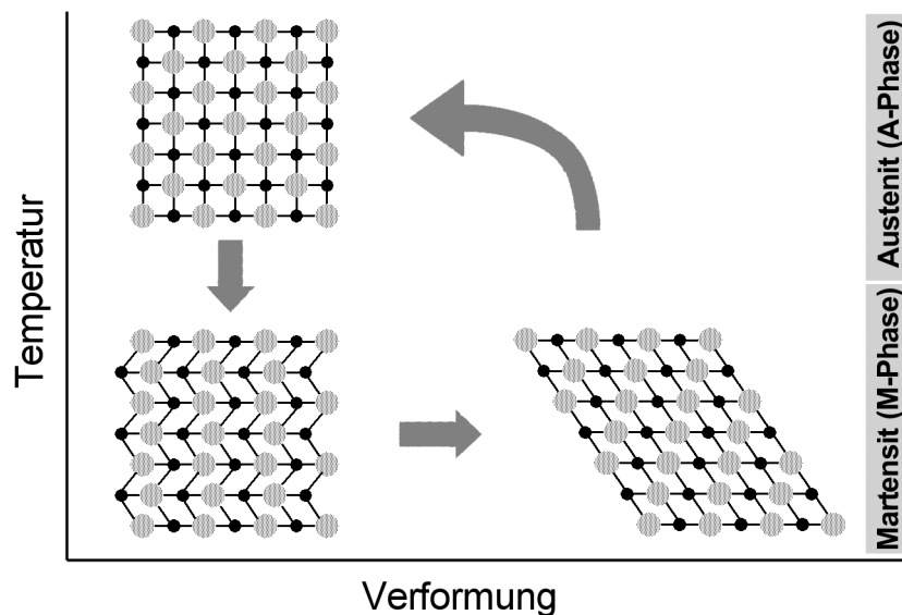
Abbildung 2.6: Martensitische Umwandlung und Formgedächtniseffekt (FGE) [6].
