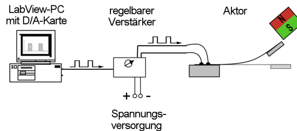
Abbildung 5.9: Schematischer Aufbau für den dynamischen Betrieb der Spiegelaktoren.
