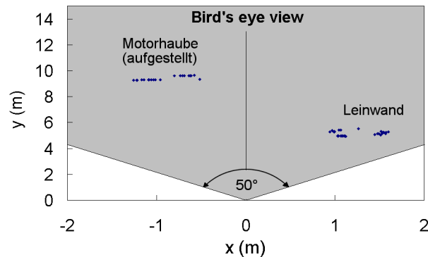
Abbildung 7.12: Abgetastete Szene mit zwei Objekten in 6 m und 9 m Abstand aus der Vogelperspektive. Die ermittelten blauen Datenpunkte liegen zunächst als Entfernung und Winkel in Polarkoordinaten vor und wurden hier in ein x–y–Diagramm übertragen.
