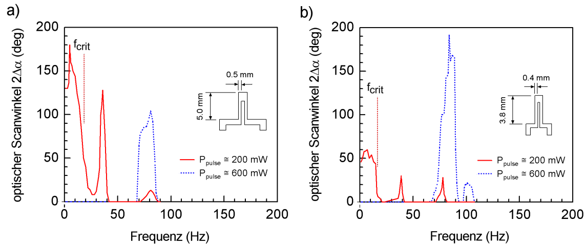
Abbildung 5.34: Scanwinkel–Frequenz–Kennlinie für Spiegelaktoren a) nach Design 2 und b) nach Design 3. Die Dicke der Verbundschicht ist in beiden Fällen gleich groß (5.5 \mu\text{m} ).
