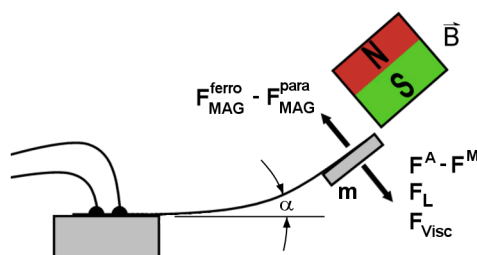
Abbildung 3.11: Im 1D-Aktorsystem aus der Formgedächtnislegierung Ni_2MnGa wirkende Kräfte. F_{MAG}^{ferro} - F_{MAG}^{para} = magnetische Kraft F_A - F_M = Formgedächtniskraft F_L = Lorentzkraft F_{Visc} = Luftreibung.
