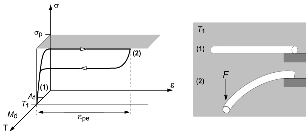
Abbildung 2.10: Spannungs-Dehnungs-Temperatur Diagramm für den pseudoelastischen Effekt.
