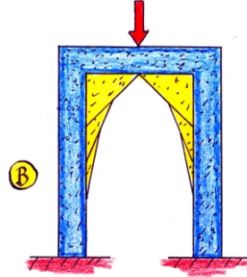
Optimierung der Ecken mit der Zugdreiecksmethode
