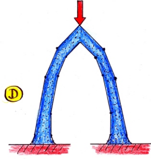
Optimierung der Kerben über den Auflagern mit der Zugdreiecksmethode
