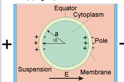
Fig. 1: Charge spatiale sur la membrane cellulaire d'une cellule sphérique.
