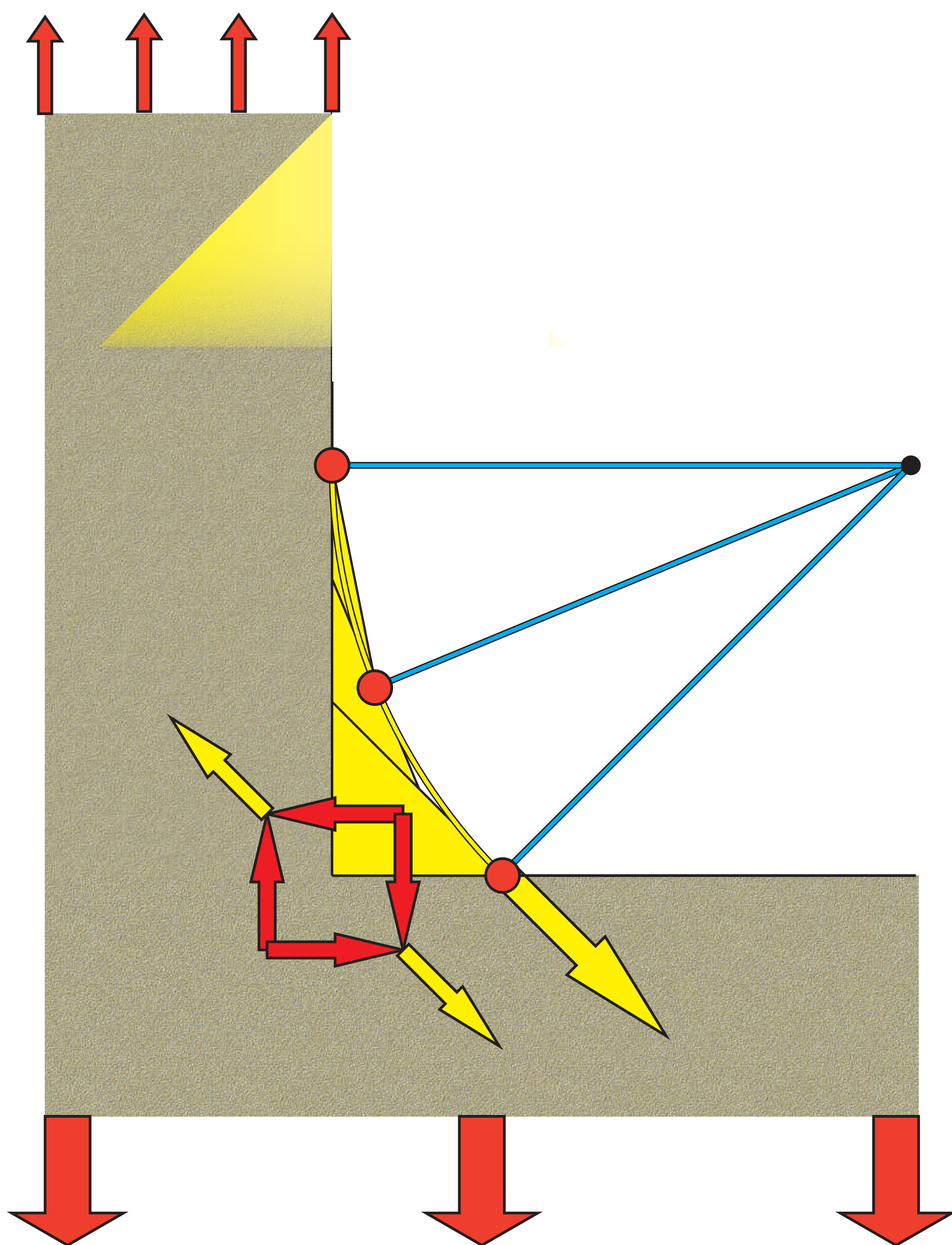
Kraftflussumlenkung mit Kraftkegelmethode
