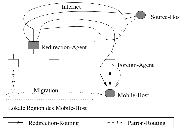
Abbildung 37. Patron-Host-Konzept.
