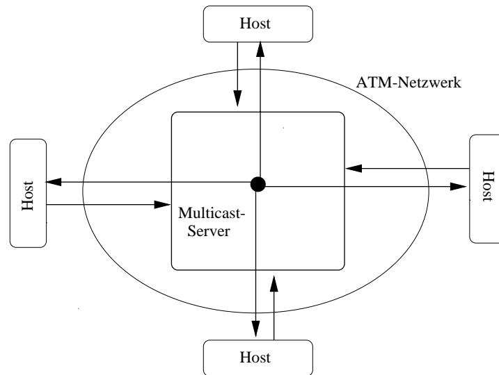
Abbildung 64. Eine Punkt-zu-Mehrpunkt-Verbindung.
