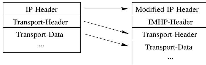
Abbildung 40. IMHP-Tunneling-Header.
