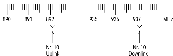
Abbildung 29. Frequenzaufteilung
