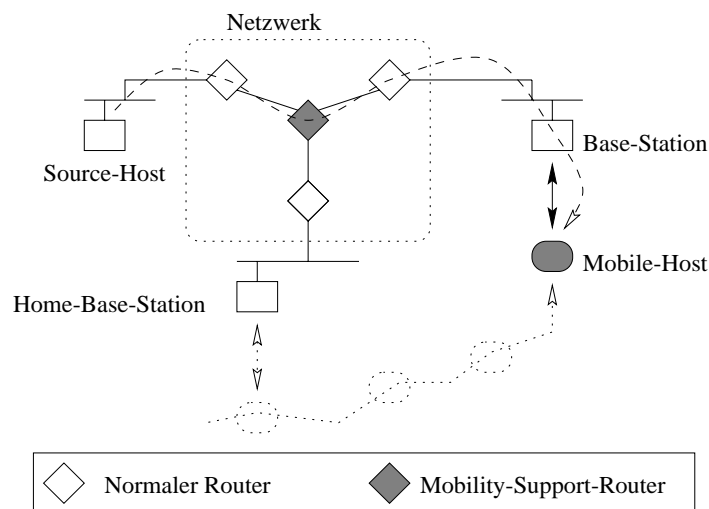
Abbildung 39. Mobility-Support-Router-Konzept.
