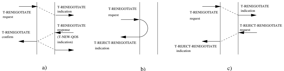
Abbildung 7. Zeitdiagramm einer a) erfolgreichen und b),c) nicht erfolgreichen Neuverhandlung
