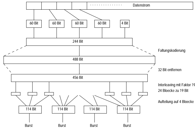
Abbildung 32. Kodierung von Nicht-Sprachdaten
