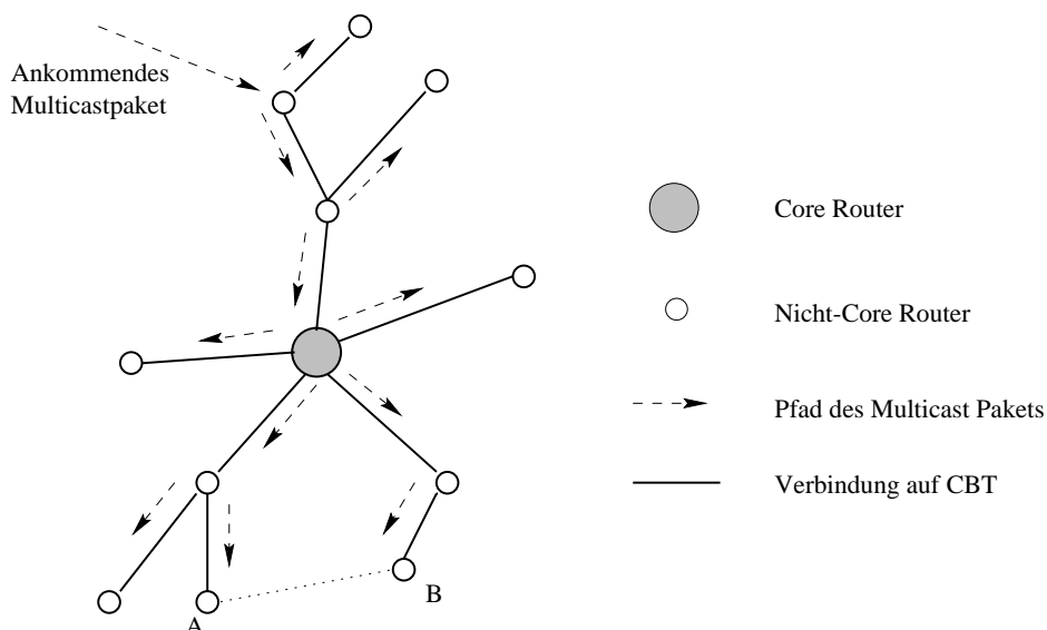
Abbildung 47. CBT Baum
