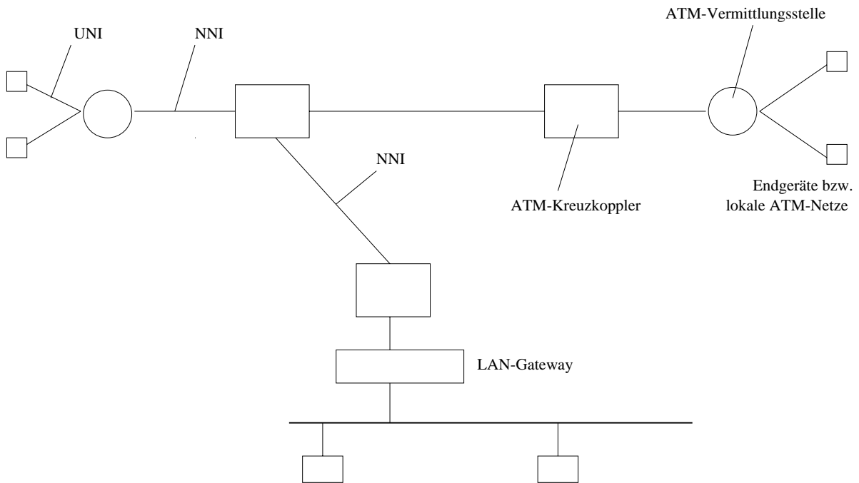
Abbildung 61. Topologische Struktur eines ATM-Netztes
