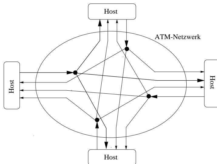
Abbildung 63. Viele Punkt-zu-Mehrpunkt-Verbindungen.
