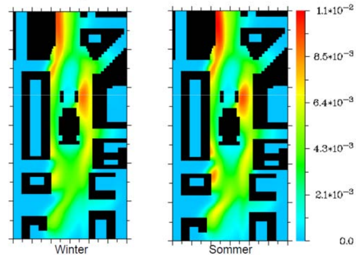
Schadstoffbelastung in 14 m Höhe Windrichtung aus 245°
