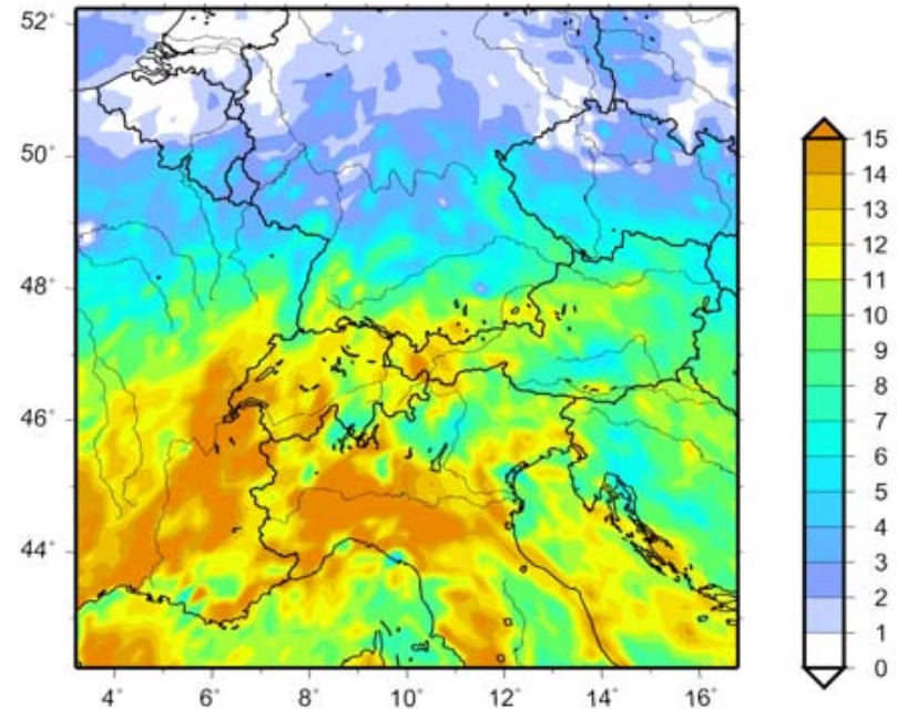
Regionale Klima-Chemie-Simulation über 2x10 Jahre mit MCCM: Zunahme der Tage mit Grenzwert- überschreitungen für bodennahes Ozon
