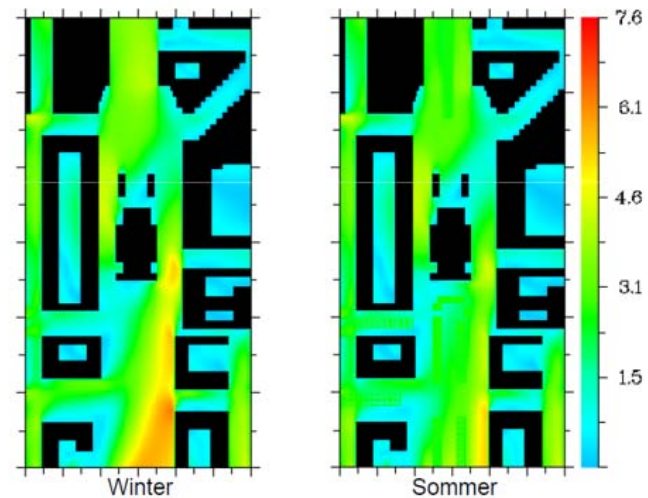
Schadstoffbelastung in 14 m Höhe Windrichtung aus 245°
