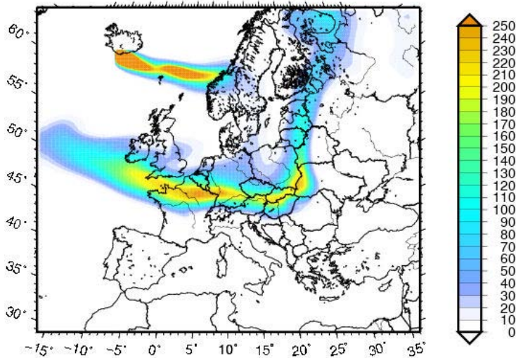
Transport einer Vulkanaschewolke
