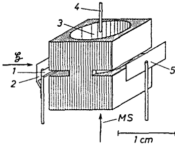
Abb. 3. Der Ionisationsdetektor: 1 = Wolframbandkathode. 2 = Abschirmblech, auf Kathodenpotential. 3 = Ionisierungsraum. 4 = Ionenauffänger. 5 = Anode. \odot = Richtung des Magnetfeldes. MS = Richtung des Molekularstrahles.
