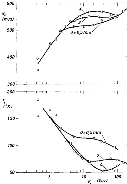
Abb. 7. Strahlgeschwindigkeit w_e und Strahltemperatur T_e von CO 2 , konvergente Düse, in Abhängigkeit vom Einlaßdruck p_0 für die Abstände d=0,5 mm, 2 mm und 4 mm.
