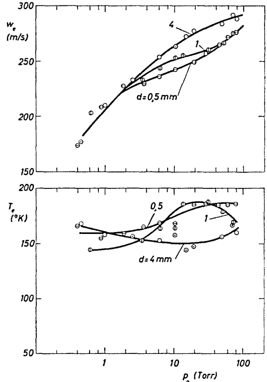
Abb. 8. Strahlgeschwindigkeit w_e und Strahltemperatur T_e von UF 6 , konvergente Düse, in Abhängigkeit vom Einlaßdruck p_0 für die Abstände d=0,5 mm, 1 mm und 4 mm.
