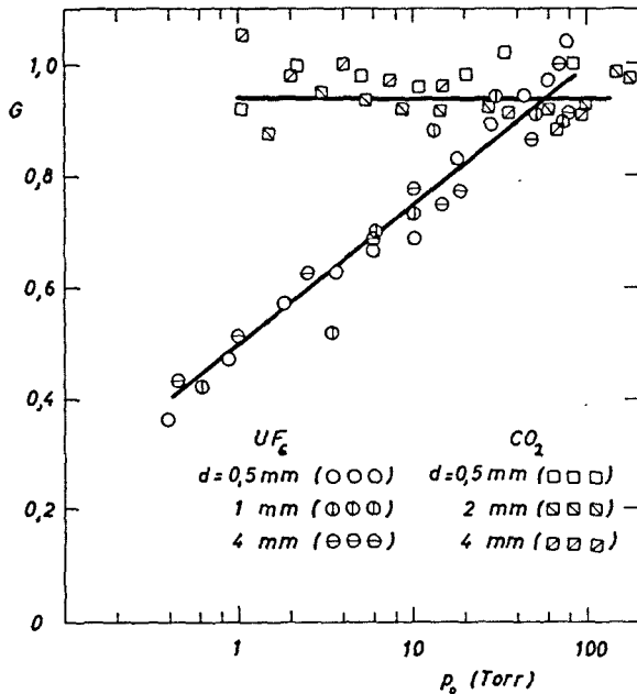
Abb. 9. Der Akkommodationsgrad G von UF_6 und CO_2 , konvergente Düse, als Funktion des Einlaßdruckes p_0 .
