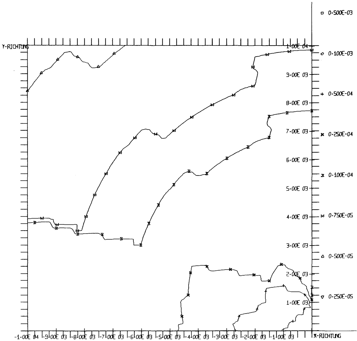
ABB-00002 ISODOSENLINIEN
