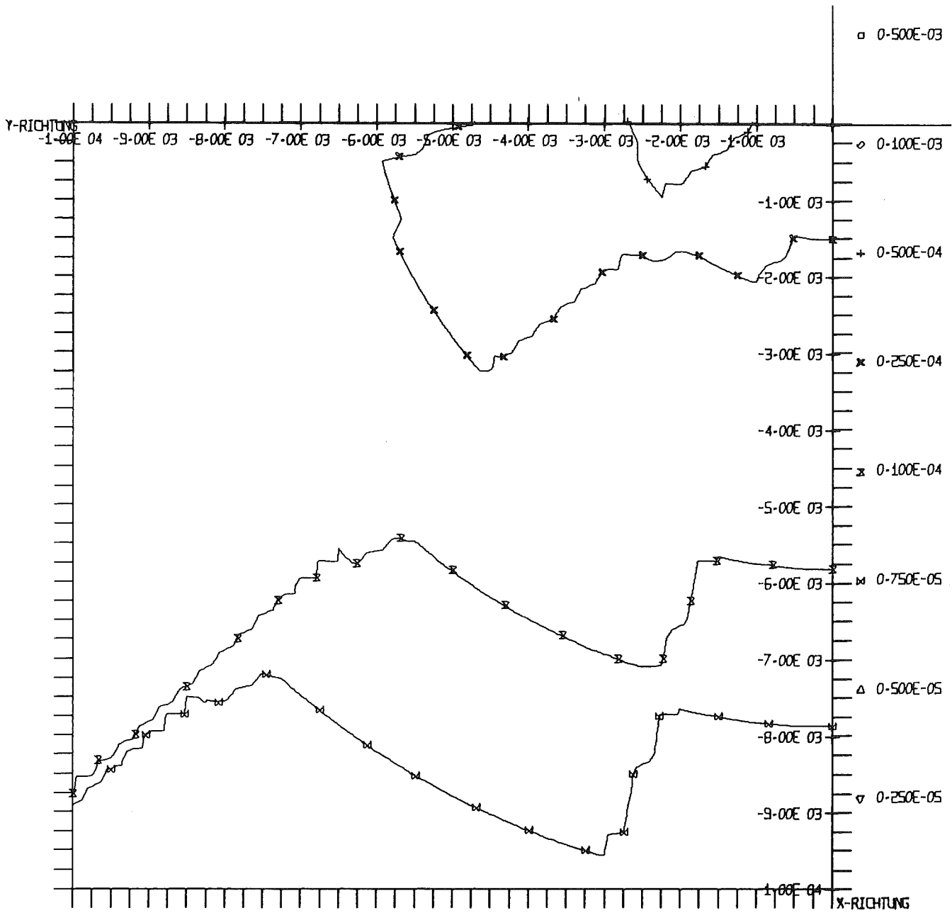
ABB-00003 ISODOSENLINIEN
