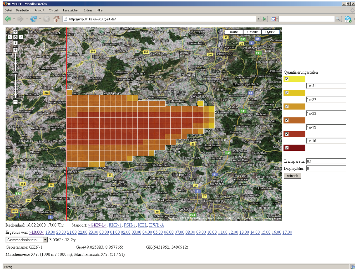
Abbildung 3: Beispiel einer RIMPUFF-Ergebnisvisualisierung im Browser unter Verwendung der Google-Maps-API für den Standort GKN-1
