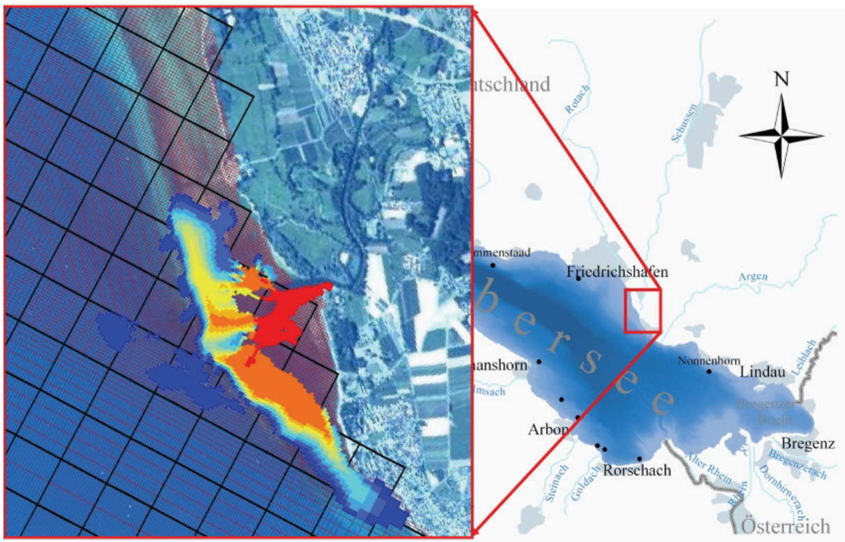
Abbildung 3: Modellnetz des großräumigen Modells (schwarz) und Lokalmmodell der Schussen mit Ausbreitung der Flusswasserfahne
