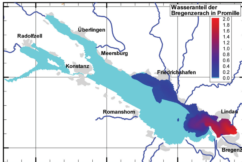
Abbildung 8: Verteilung des Wassers aus der Bregenzerrach an der Seeoberfläche 4 Tage nach einem potenziellen Ölunfall am 02.07.2007 in der Bregenzerrach
