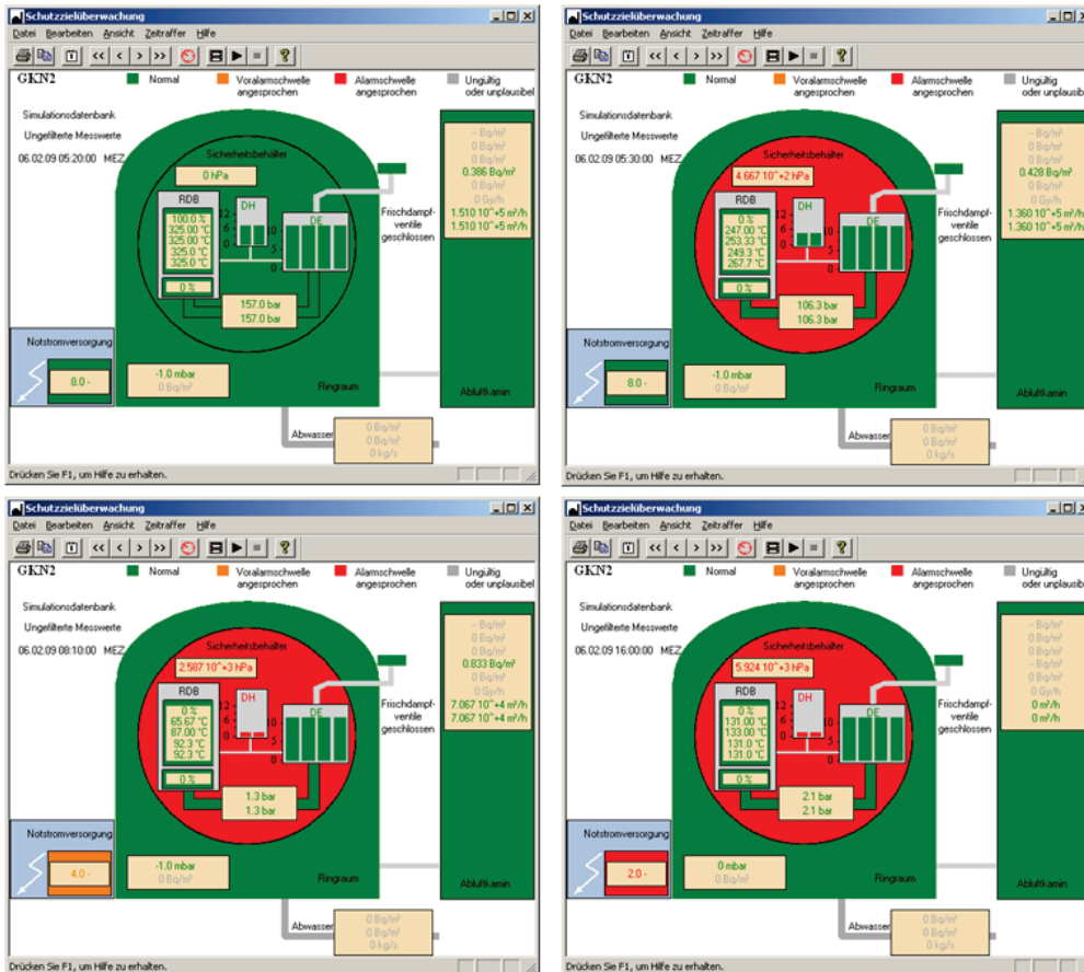
Abbildung 5: Schutzzielschaubild GKN-2 im Verlauf der Simulation: Ausgangslage (oben links); nach Leckage im Primärkreis kontinuierlich ansteigender Druck (von oben rechts bis unten rechts); Beginn Ausfall Notstromversorgung (unten links); bis kurz vor Übungsende waren laut Szenario nur 2 Notstromschienen verfügbar. Das Containment hatte nicht versagt.
