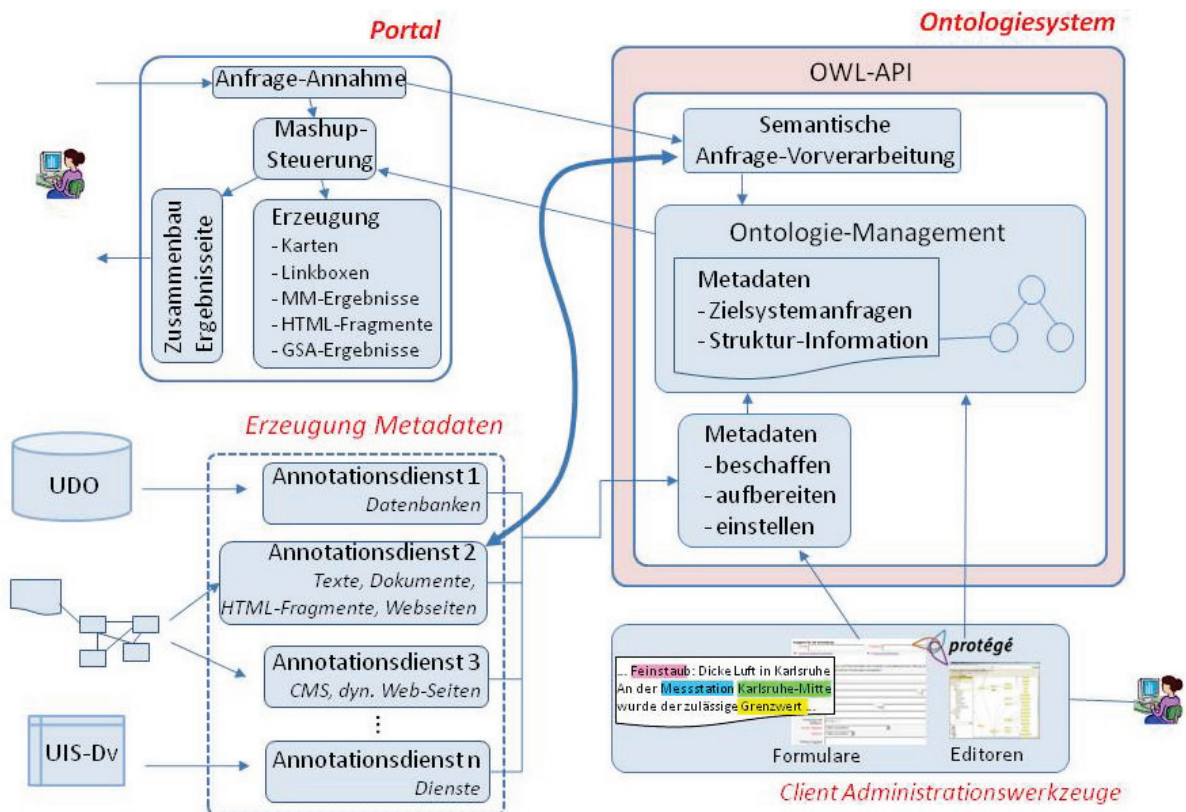
Abbildung 3: Erweiterte Architektur des Gesamtsystems
