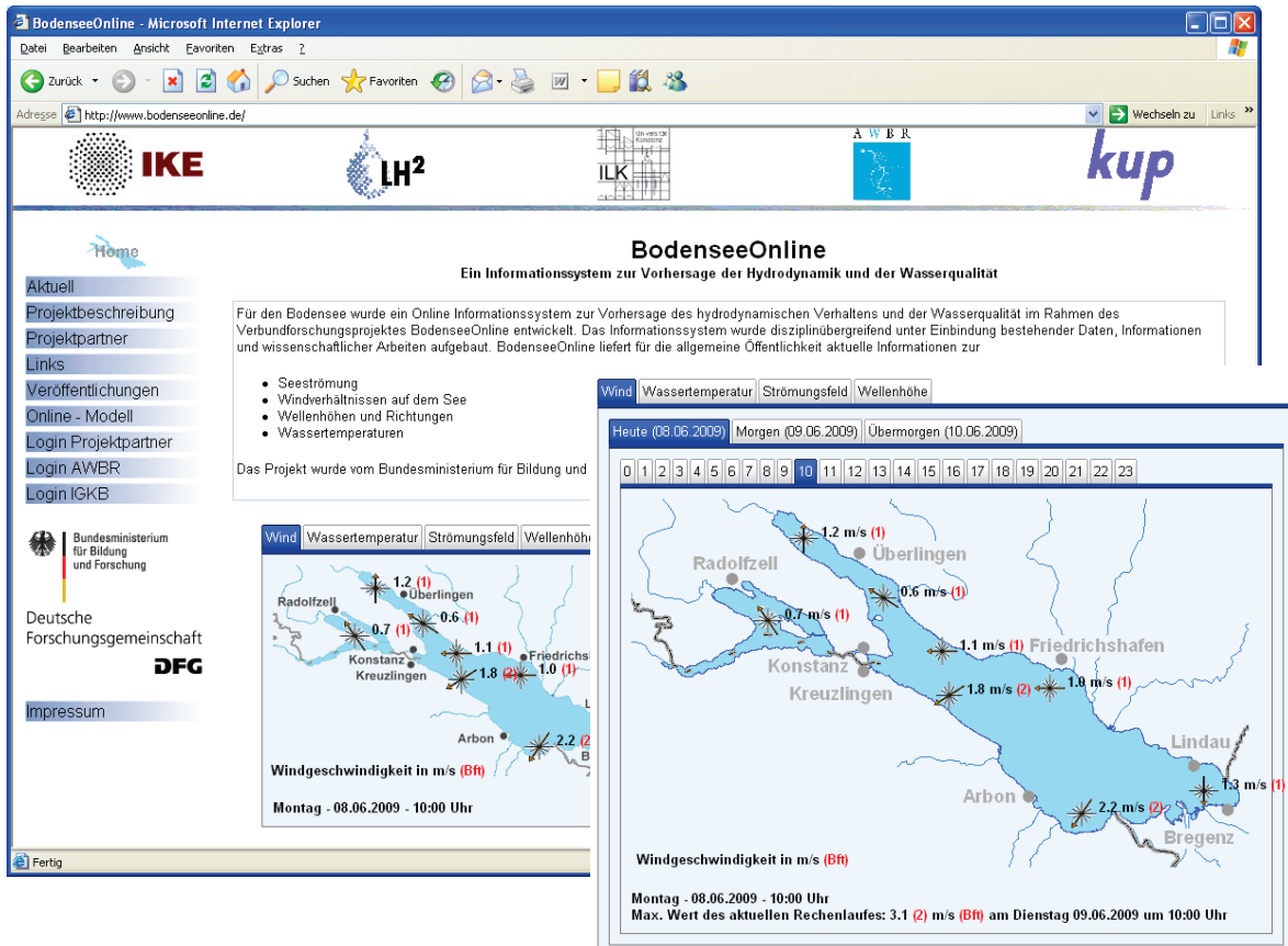
Abbildung 3: Informationen aus BodenseeOnline zu den Wind-, Temperatur-, Wellen- und Strömungsverhältnissen für die Öffentlichkeit
