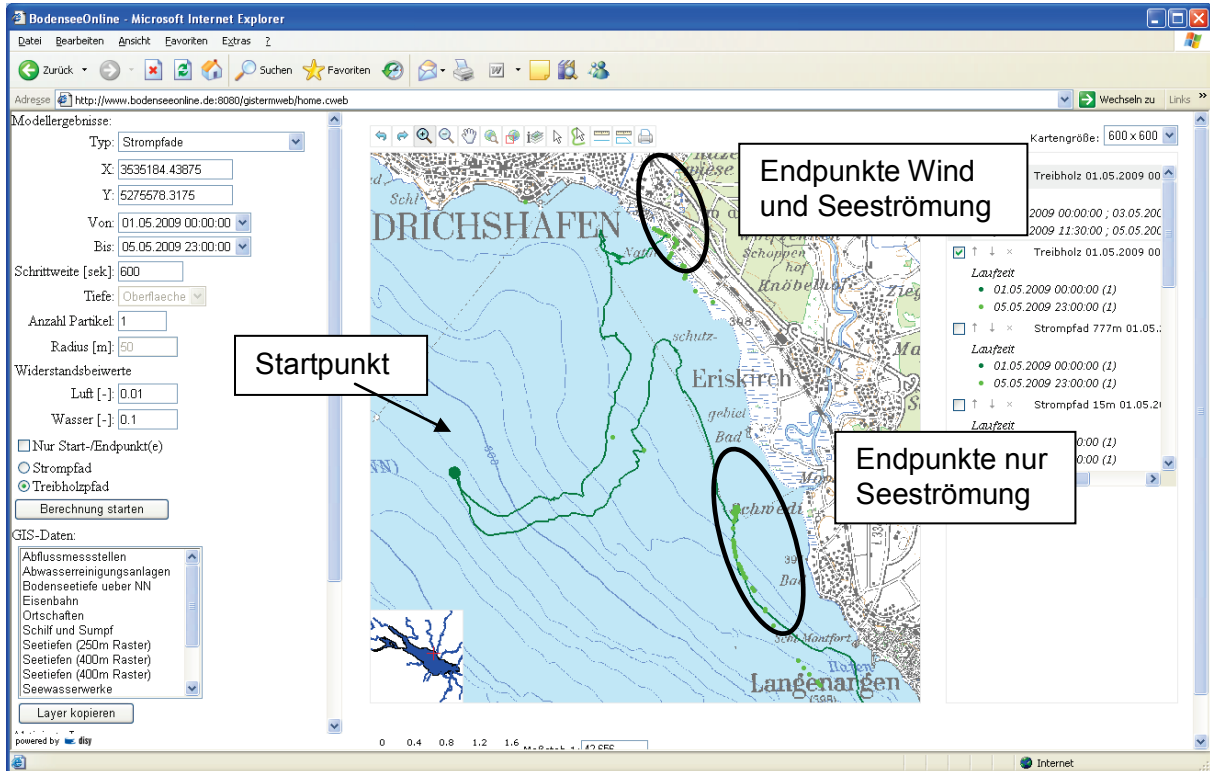
Abbildung 5: Bewegung von Partikeln an der Seeoberfläche aufgrund der Seeströmung und in Kombination mit dem Windfeld in GISTerm Web
