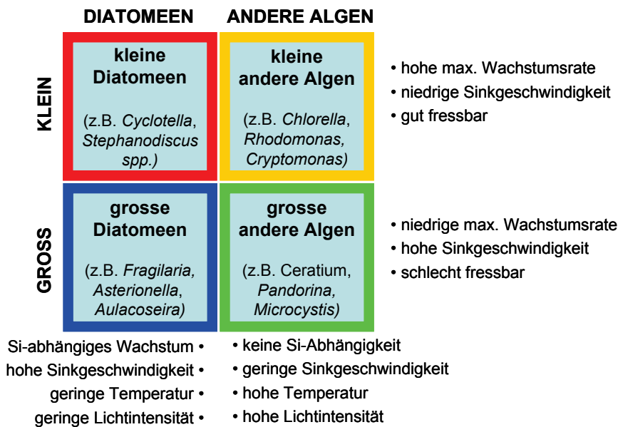
Abbildung 2: Funktionelle Klassifikation des Phytoplanktons in vier Typgruppen
