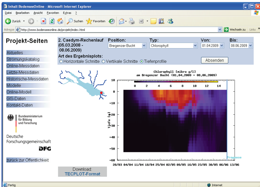
Abbildung 7: Tiefenprofil der Chlorophyllkonzentration in der Bregenzener Bucht
