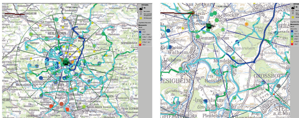
Abbildung 6: Darstellung NBR-Spuren und REI-Messungen von Betreiber, LUBW und ABC-Erkundern: Übersicht (links) und südliche Zentral- und Mittelzonen (rechts).
