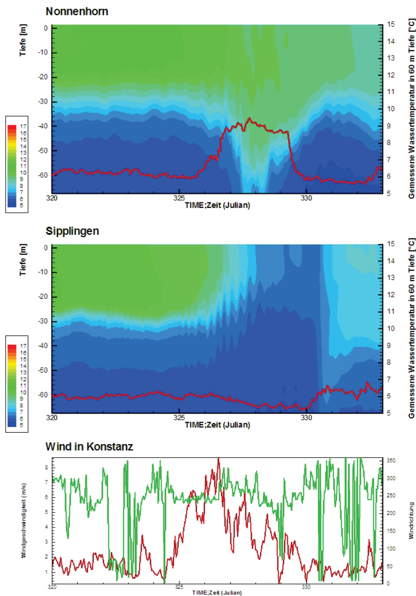
Abbildung 8: Oben: gemessene Temperatur in Nonnenhorn in 60 m Tiefe (rote Linie) und berechnetes Temperaturprofil in Nonnenhorn. Mitte: gemessene Temperatur in Sipplingen in 60 m Tiefe (rote Linie) und berechnetes Temperaturprofil in Sipplingen. Unten: gemessene Windgeschwindigkeit (rote Linie) und Windrichtung (grüne Linie) in Konstanz
