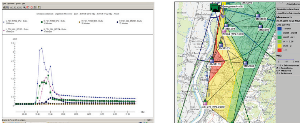
Abbildung 4: Simulation der Immissionsdaten (Halbring auf deutscher Seite); Zeitreihe (links) und Isofläche (rechts).
