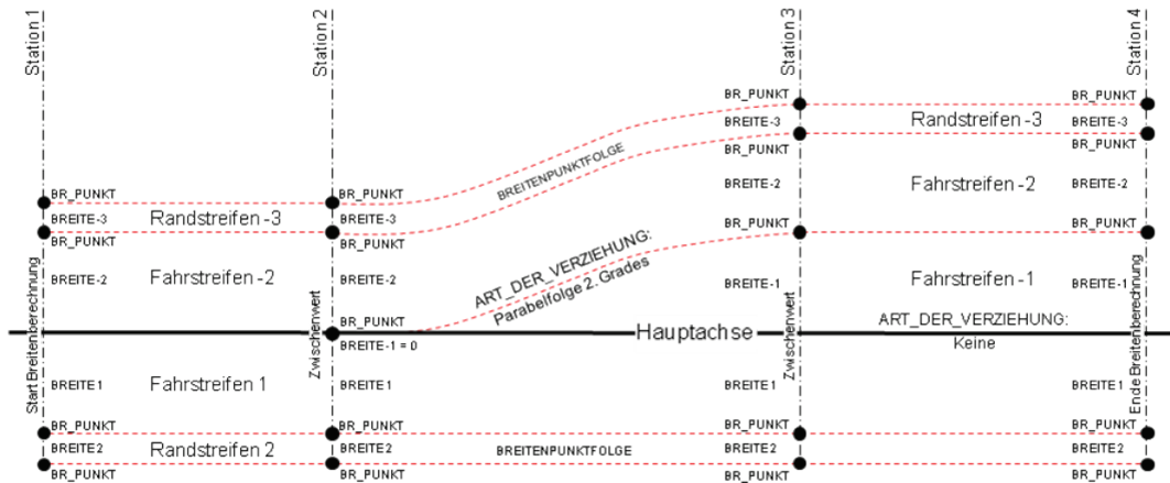
Abbildung 4: Exemplarisches Deckenbuch nach der Modellierung des OKSTRA®
