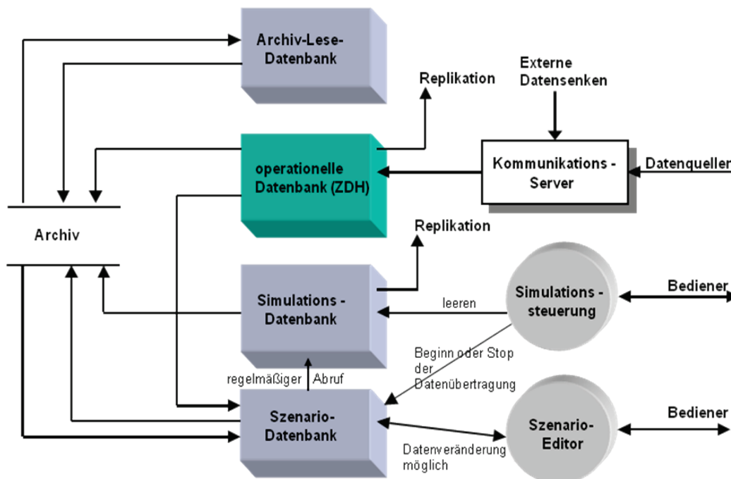
Abbildung 1: Übersicht über die verschiedenen KFÜ-Datenbanken
