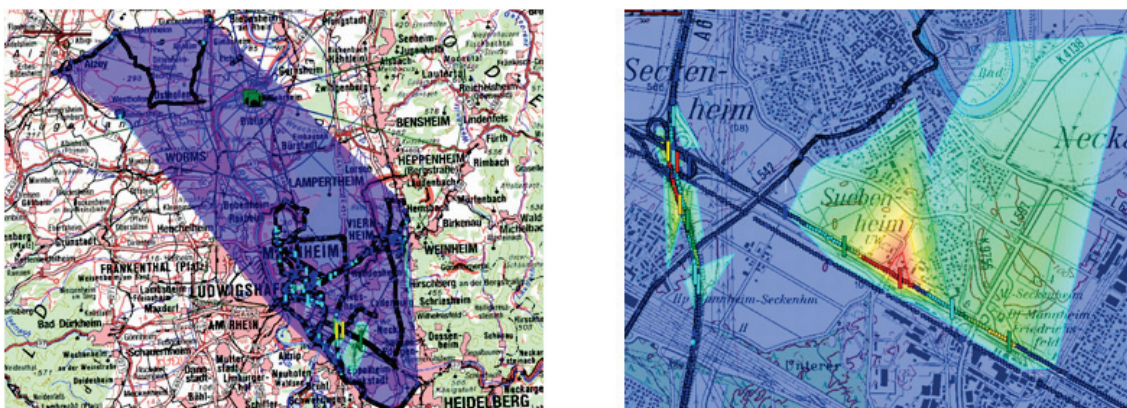
Abbildung 2: Natural Background Reduction (NBR)-Messungen verschiedener ABC-Erkunder aus Rheinland-Pfalz und Baden-Württemberg. Die rechts im Stadtgebiet von Mannheim erkennbaren Erhöhungen gehen auf den Einsatz künstlicher Strahlenquellen zurück.
