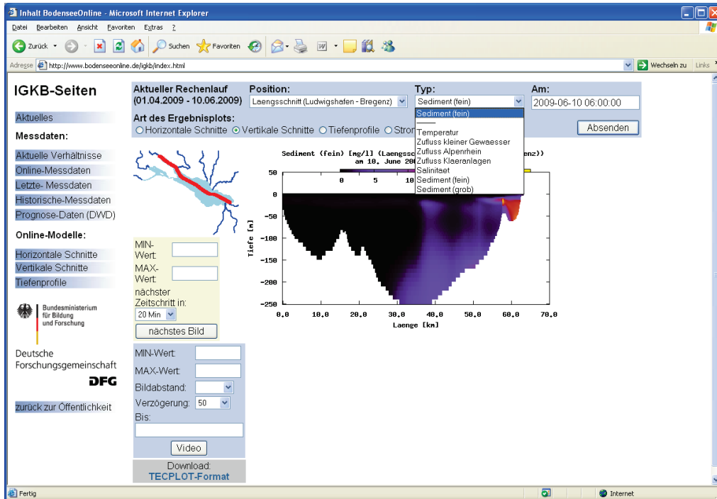
Abbildung 6: Vertikale Verteilung der Sedimentkonzentration entlang der Seelängsachse
