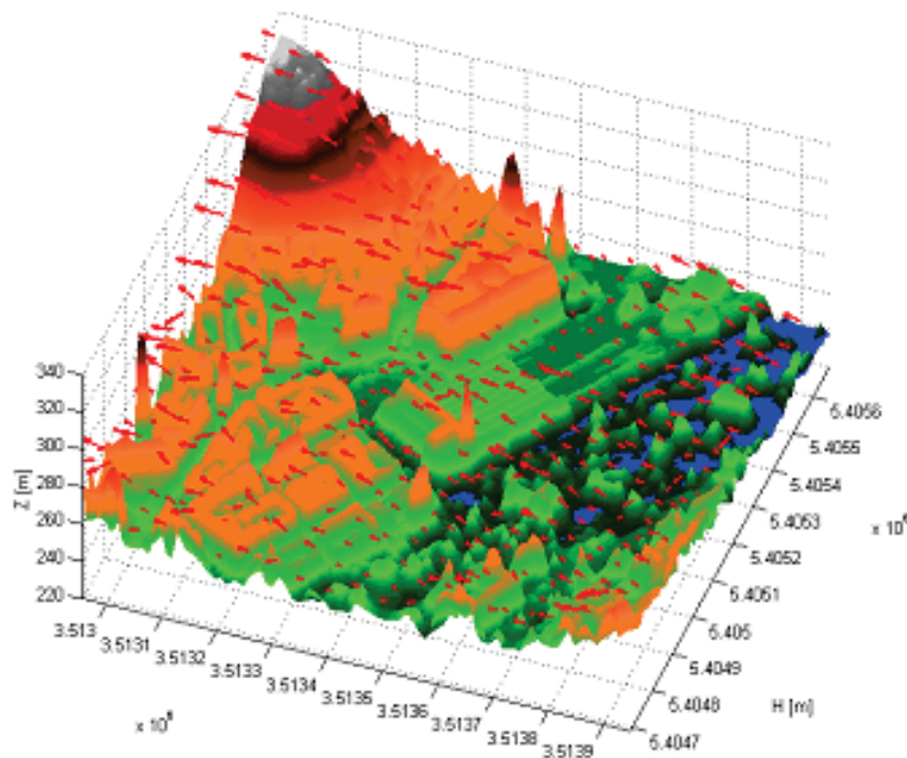
Abbildung 4: Topographie des Modellgebiets und herrschende Windverhältnisse
