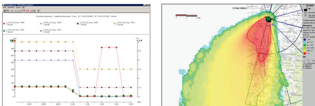
Abbildung 3: Wetterprognose mit vorhergesagter Winddrehung und sich daraus ergebende ABR-Prognose
