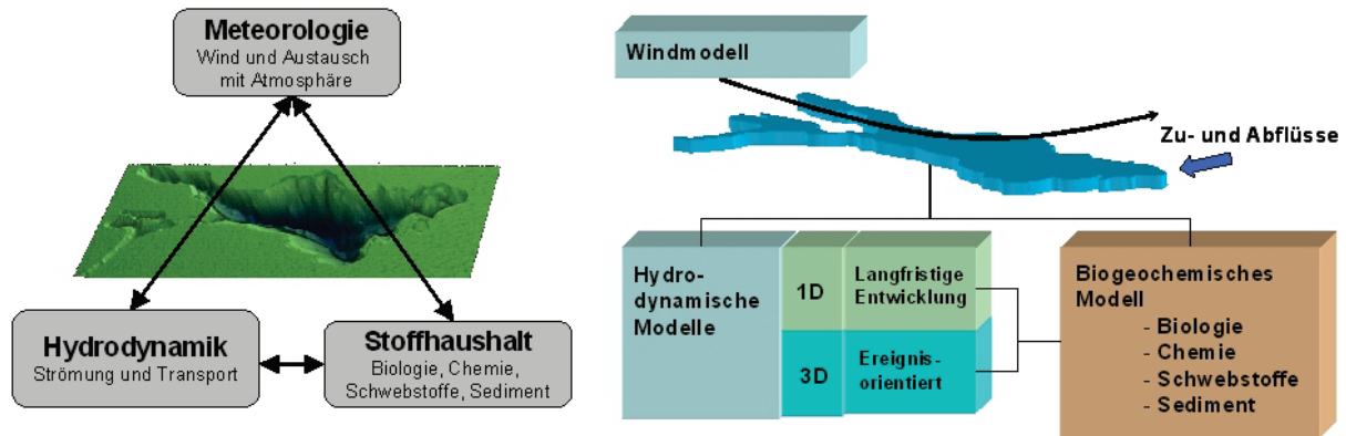
Abbildung 1: Prozesse und Antriebsgrößen (links), Modellsystem von BodenseeOnline (rechts)
