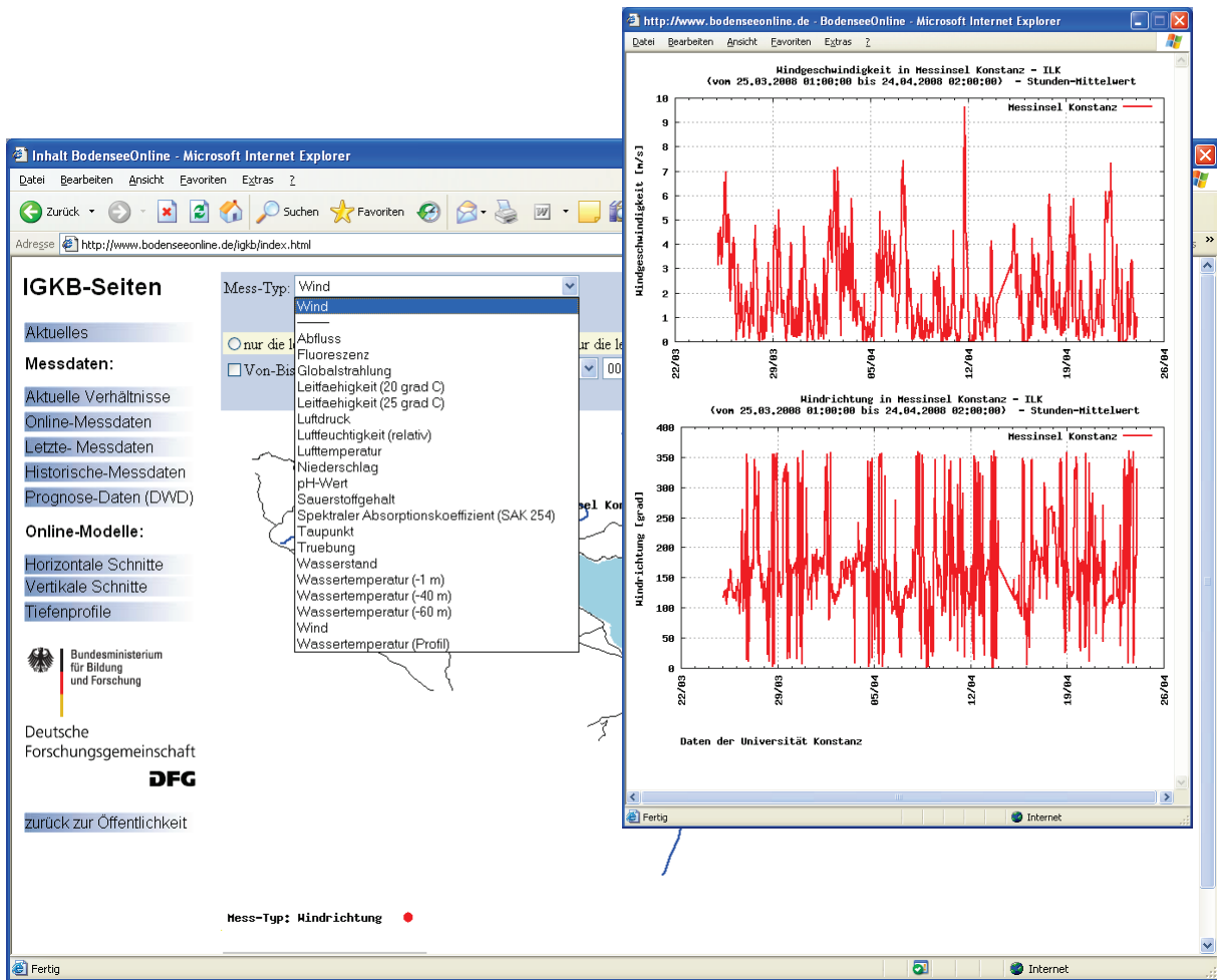
Abbildung 4: Auswertung von Online-Messdaten mit Hilfe von BodenseeOnline
