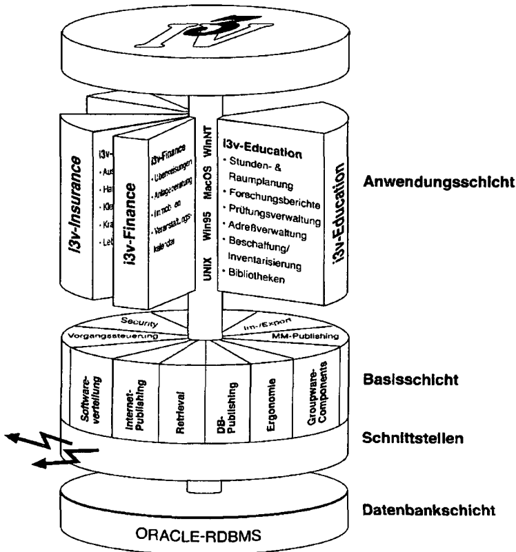
Abb. 2: i3v-Architektur
