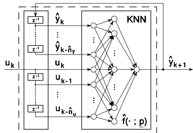
Abb. 1: Dynamisches Modell bestehend aus Künstlichem Neuronale Netz zur Approximation der Nichtlinearität und einem vorgeschalteten Block mit Zeitverzögerungen.
