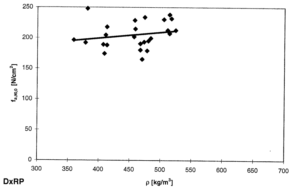
Abb. D-14: Nageltragfähigkeit-Rohdichte-Abhängigkeit der Reihen D-RP
