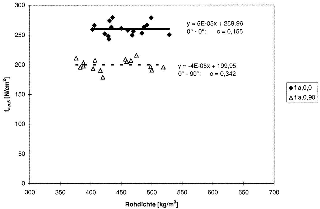
Abb. D-28: Umgerechnete Nageltragfähigkeitswerte in Abhängigkeit von der Rohdichte für Nagelplatte E
