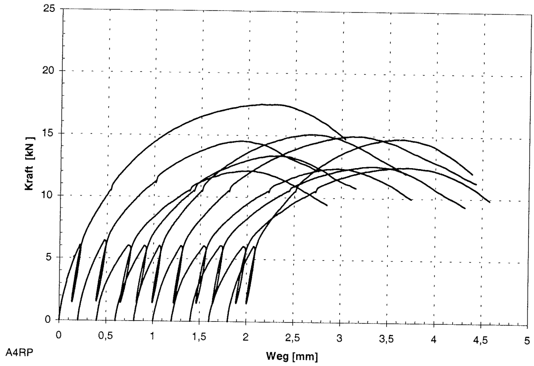
Abb. C-8: Last-Verschiebungs-Diagramm der Reihe A4RP
