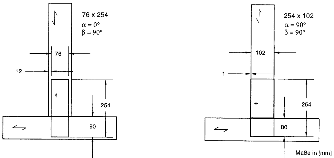
Abb. A-9: Form und Abmessungen der Versuchskörper der Reihe D
