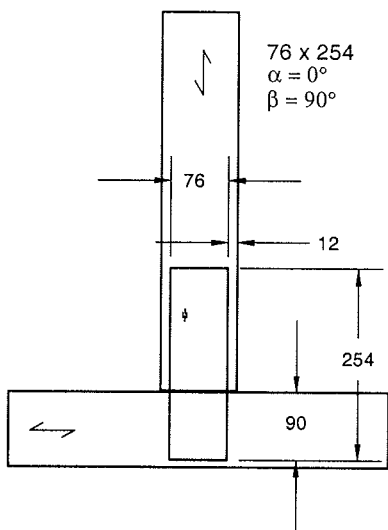
Abb. A-7: Form und Abmessungen der Versuchskörper der Reihe B
