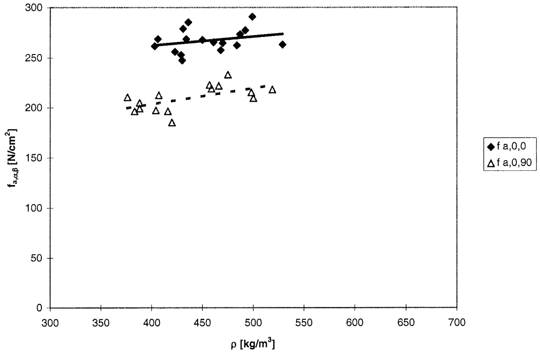
Abb. D-27: Vergleich der Abhängigkeiten für Nagelplatte E
