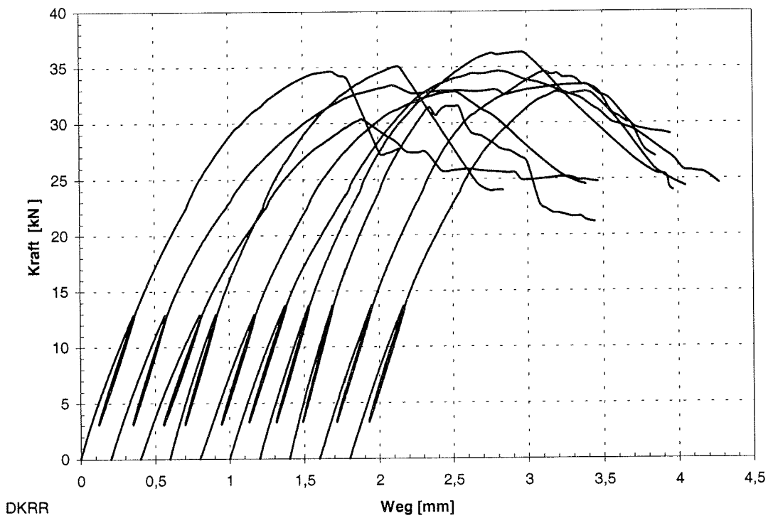
Abb. C-66: Last-Verschiebungs-Diagramm der Reihe DKRR
