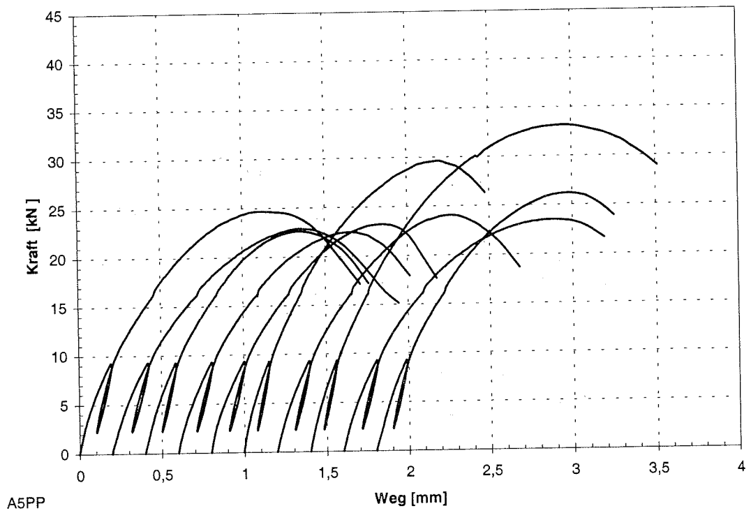
Abb. C-4: Last-Verschiebungs-Diagramm der Reihe A5PP
