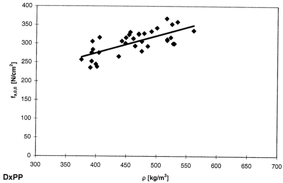
Abb. D-13: Nageltragfähigkeit-Rohdichte-Abhängigkeit der Reihen D-PP
