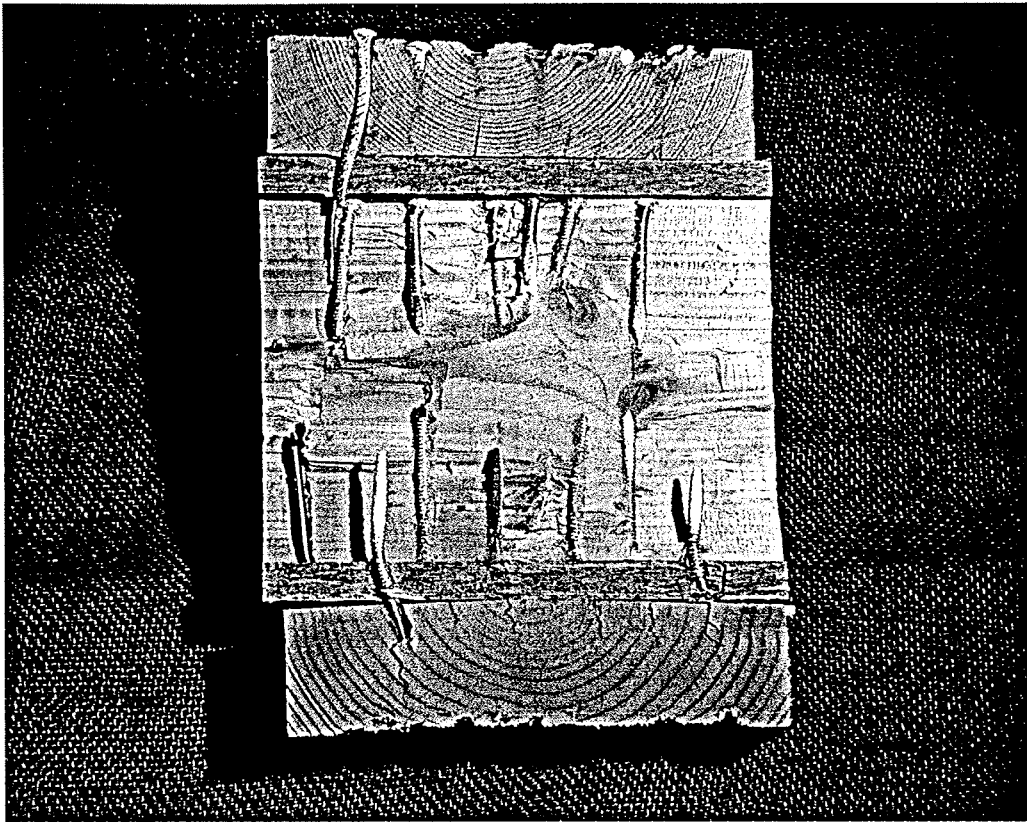
Bild A7: Aufgespaltener Versuchskörper
